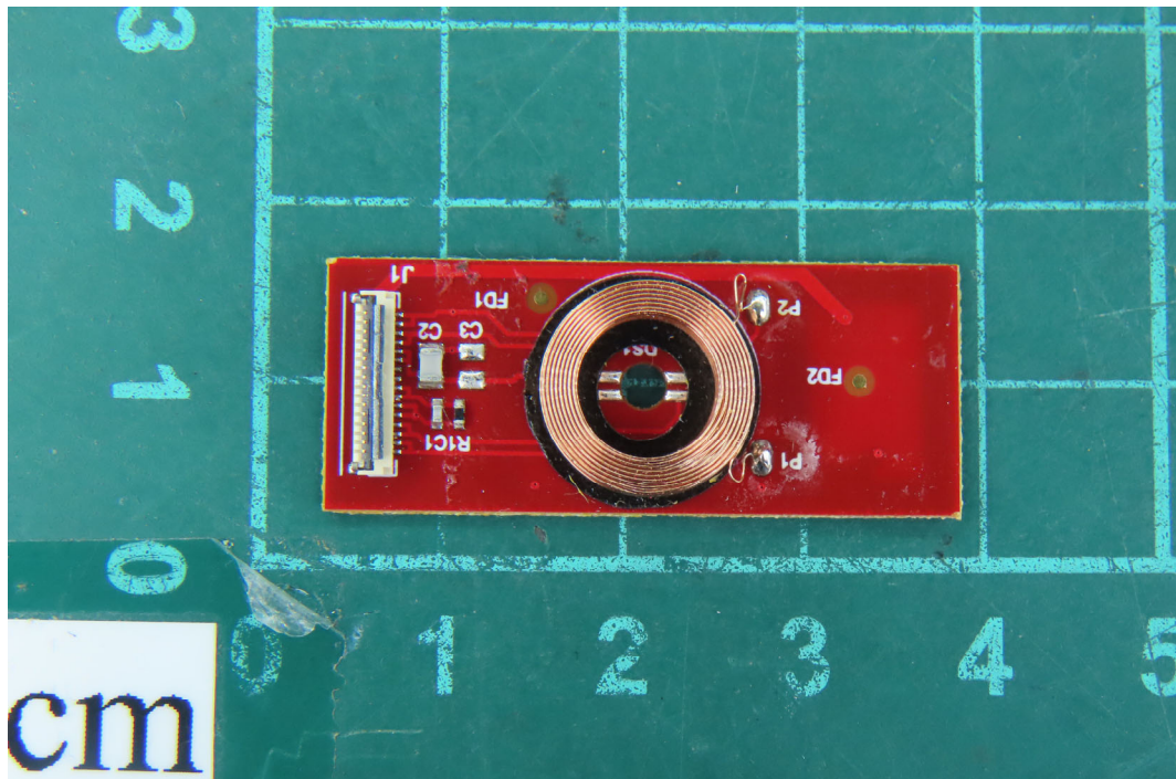
(40) EUT Photo
