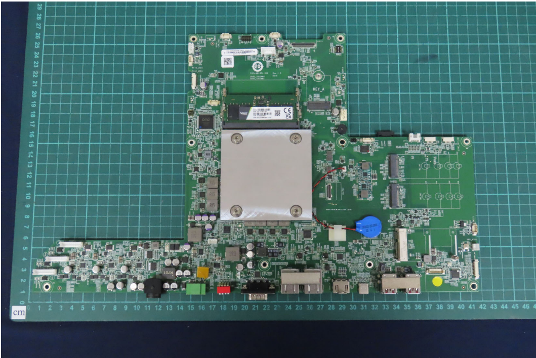
(69) EUT Photo
