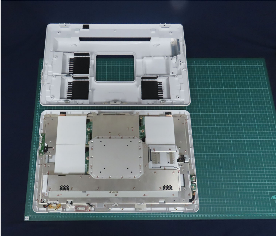
(87) EUT Photo
