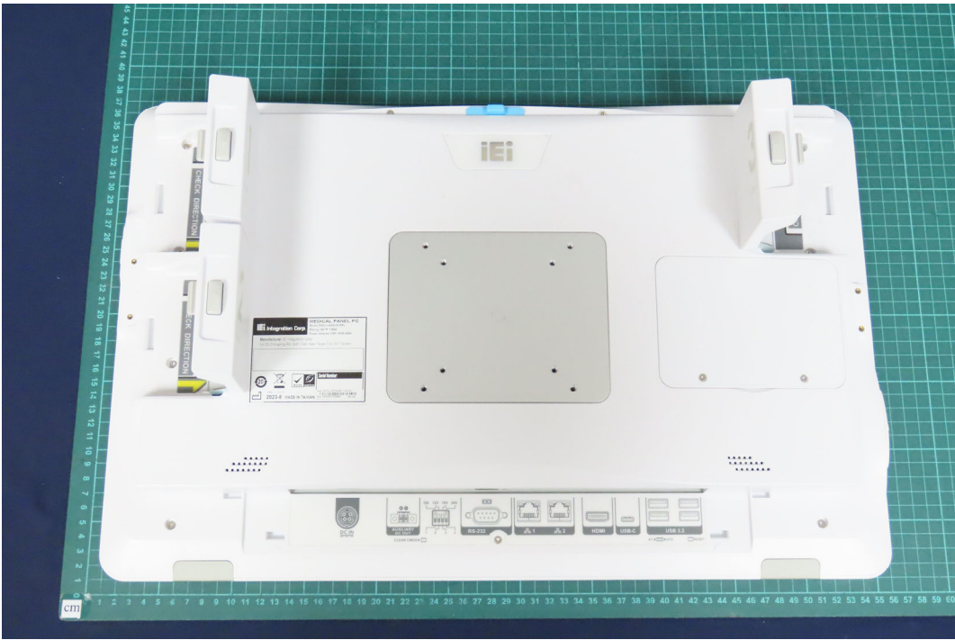
(86) EUT Photo
