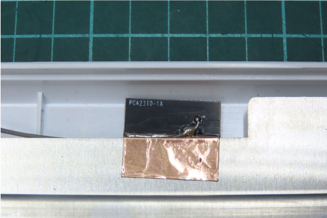
(75) EUT Photo
