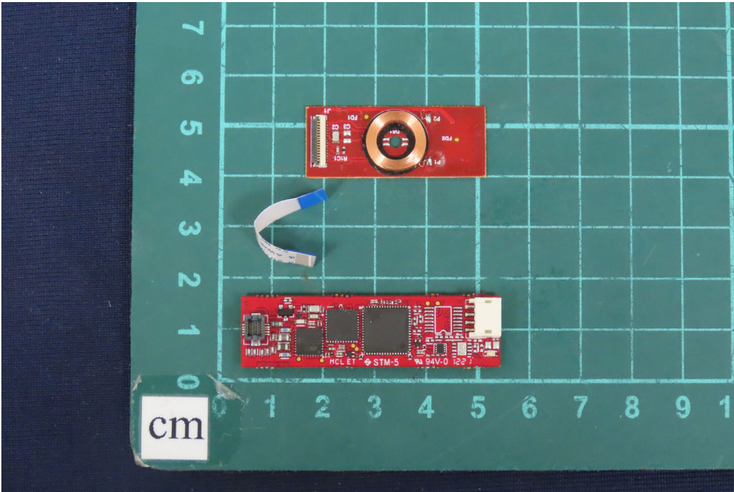
(119)EUT Photo
