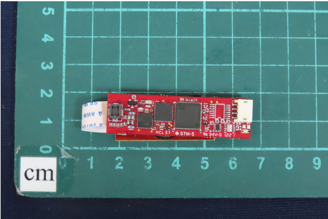
(118)EUT Photo
