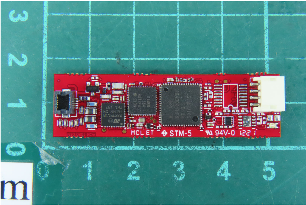
(120)EUT Photo
