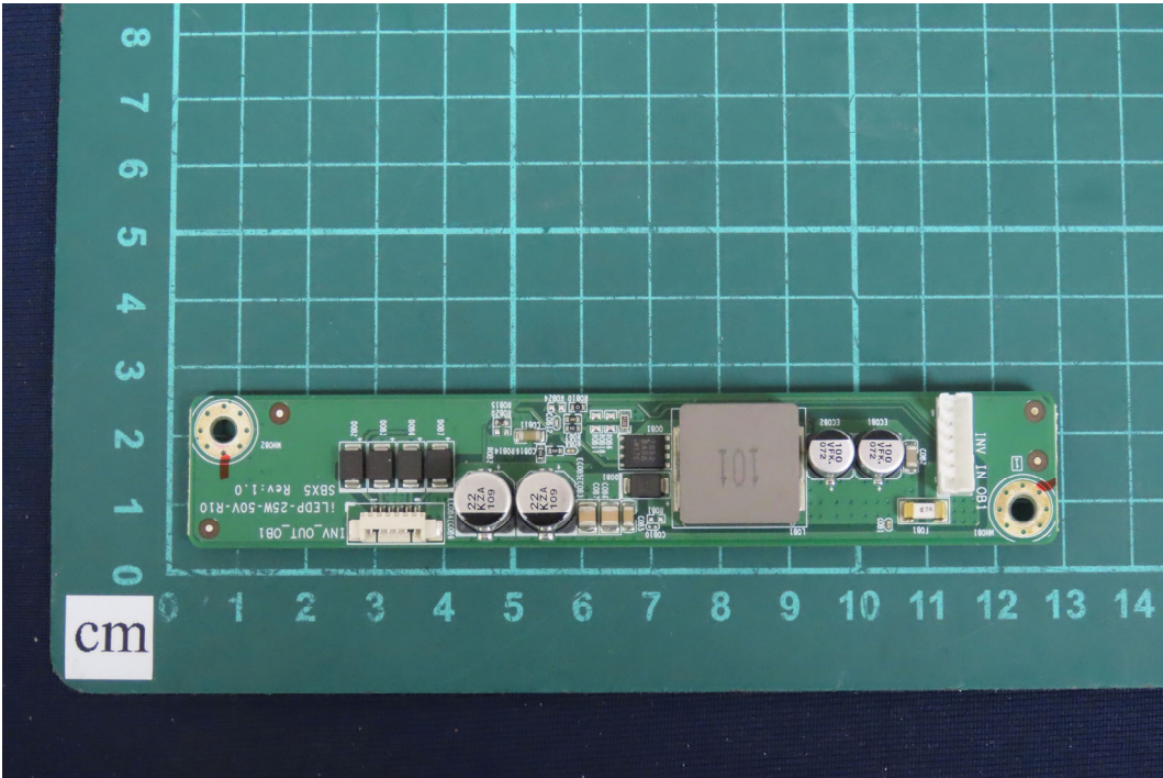
(139)EUT Photo
