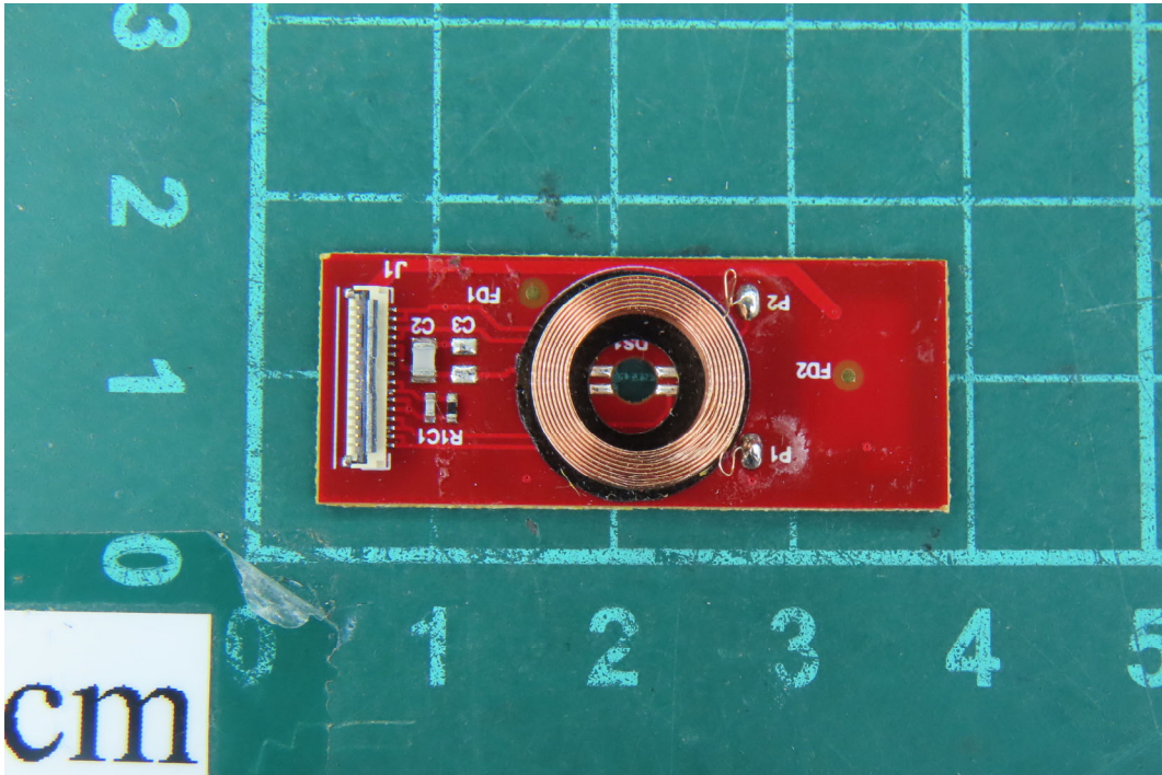
(163)EUT Photo
