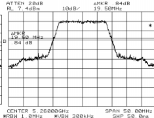
302(20 dB BW)
