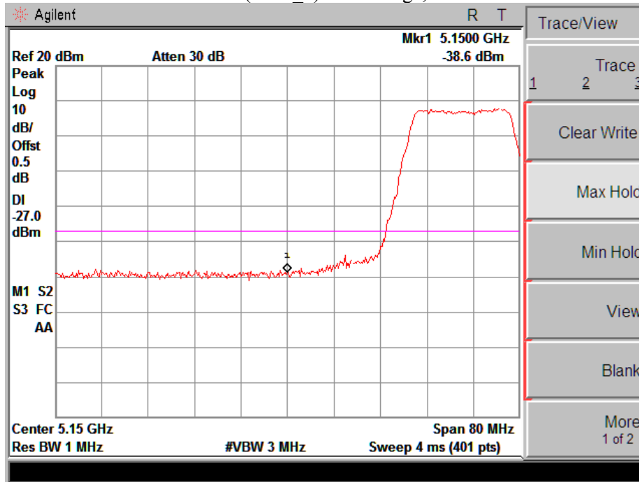
TX Mode (ANT_4): Band Edge, Left Side
