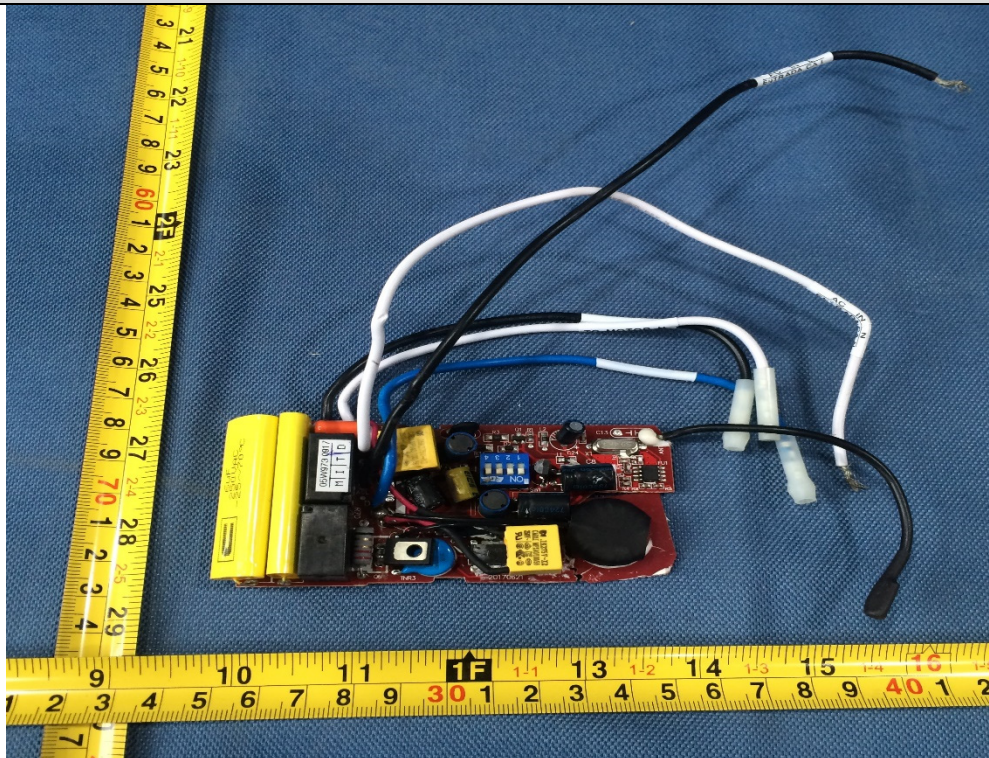
EUT Photo
