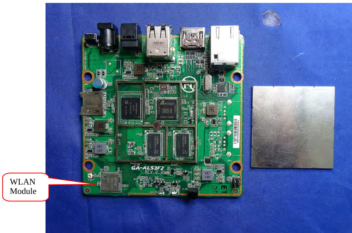
(10) EUT Photo
