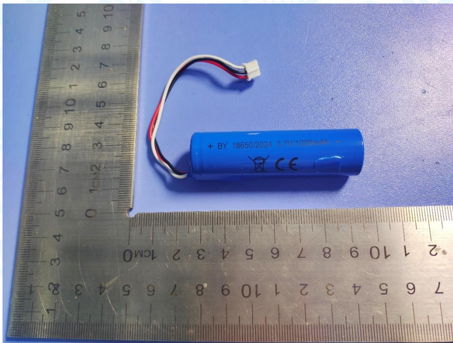
Photo 14 Battery parameters
