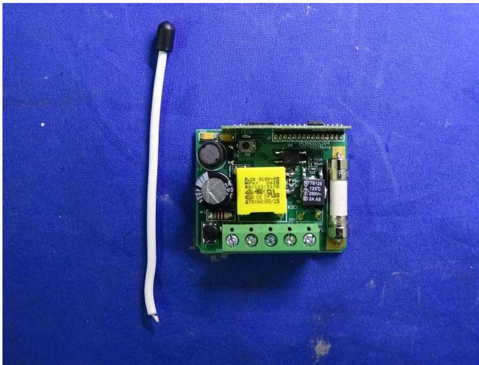
(10) EUT Photo
