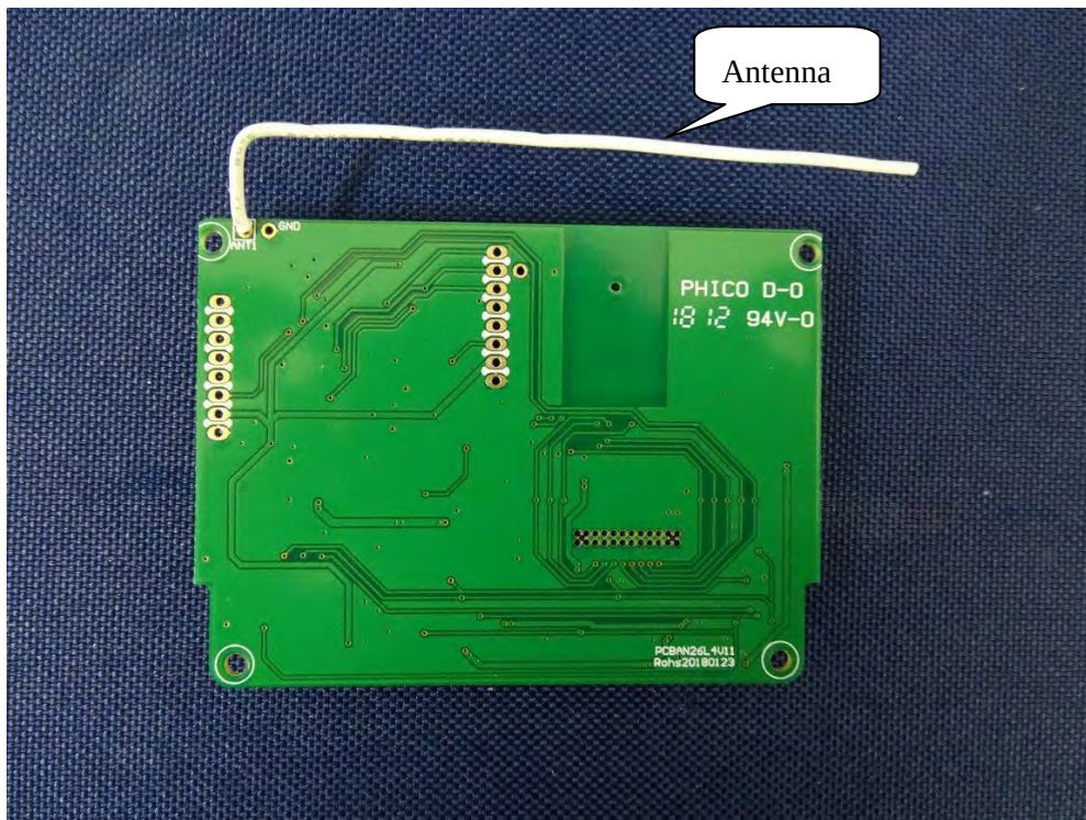
(36) EUT Photo
