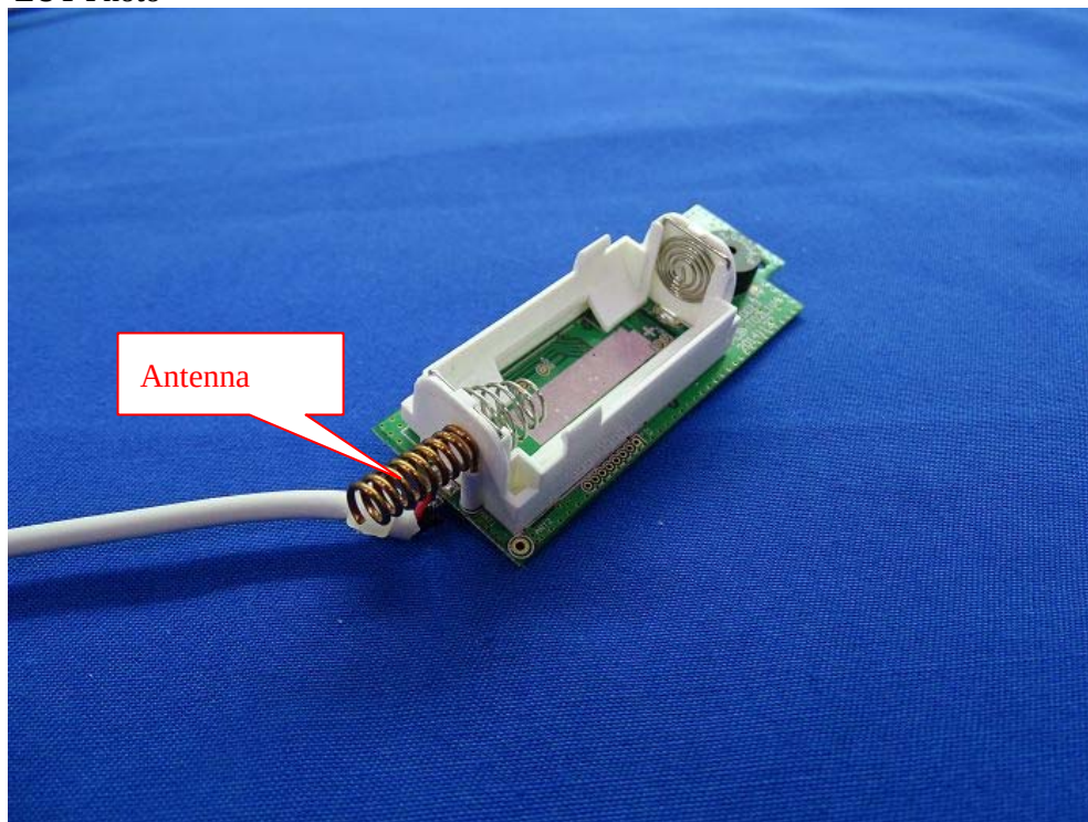
(41) EUT Photo
