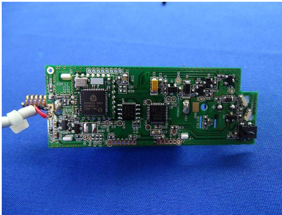
(16) EUT Photo
