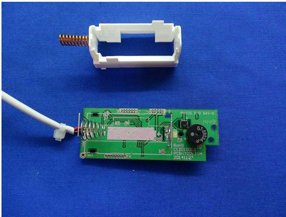
(14) EUT Photo
