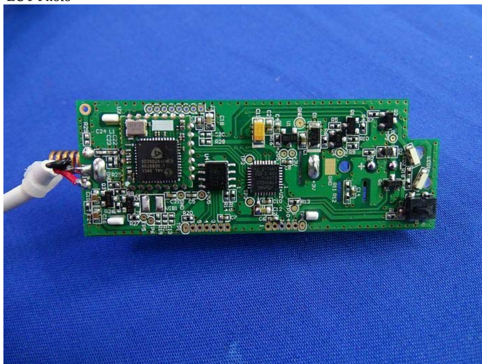
(44) EUT Photo
