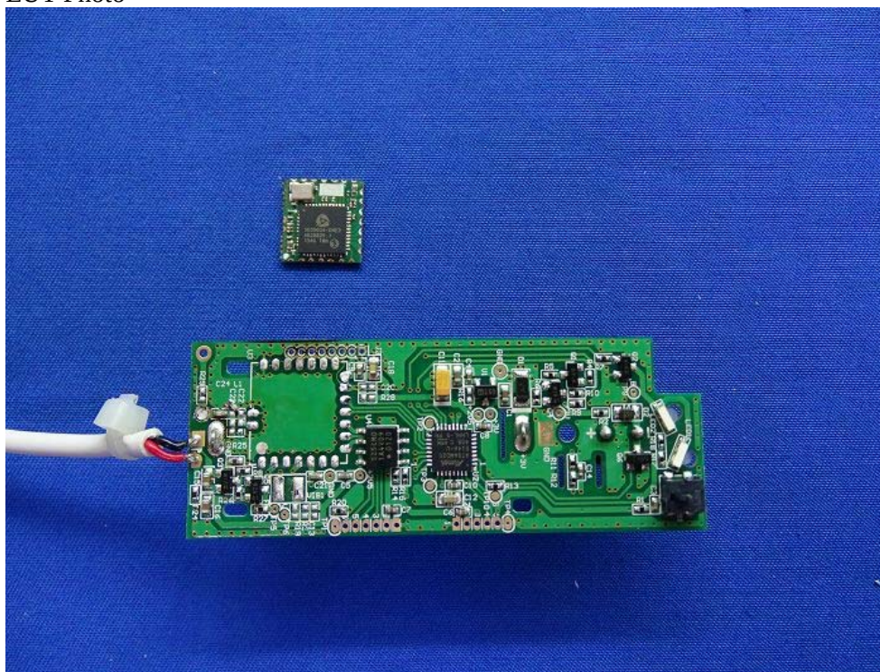
(17) EUT Photo
