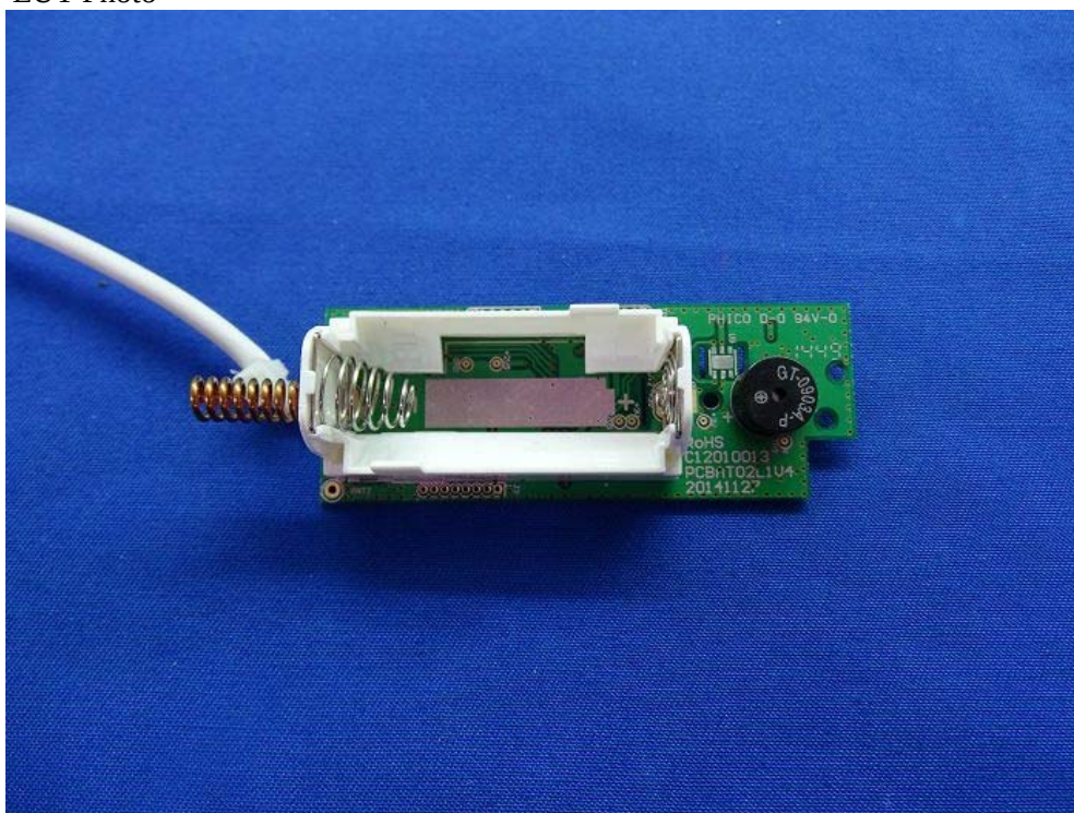
(40) EUT Photo
