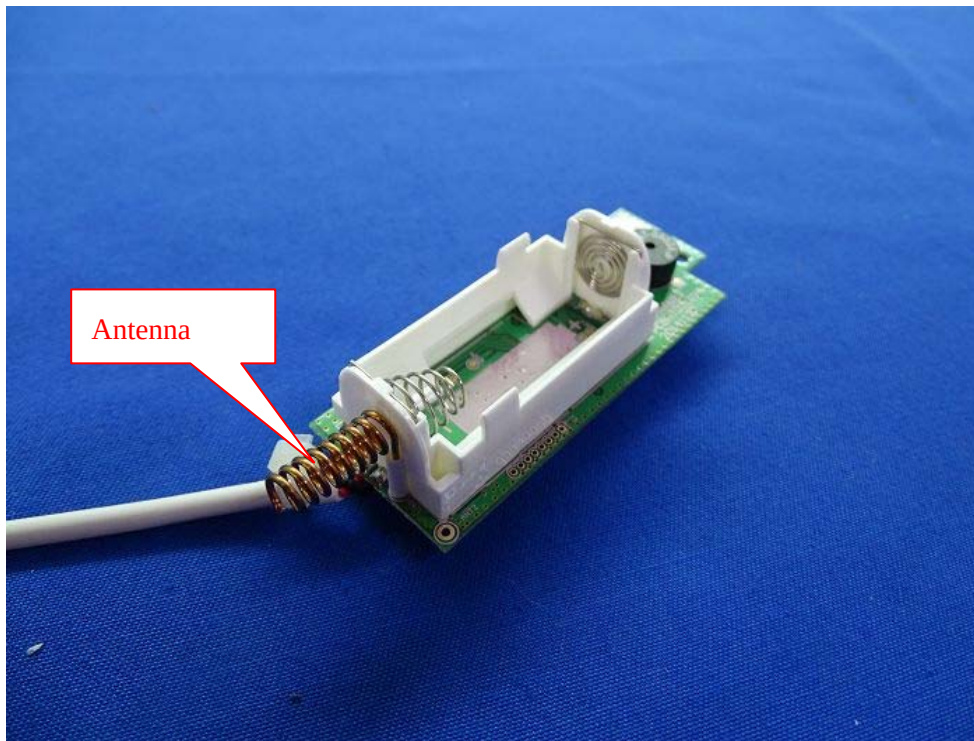
(12) EUT Photo
