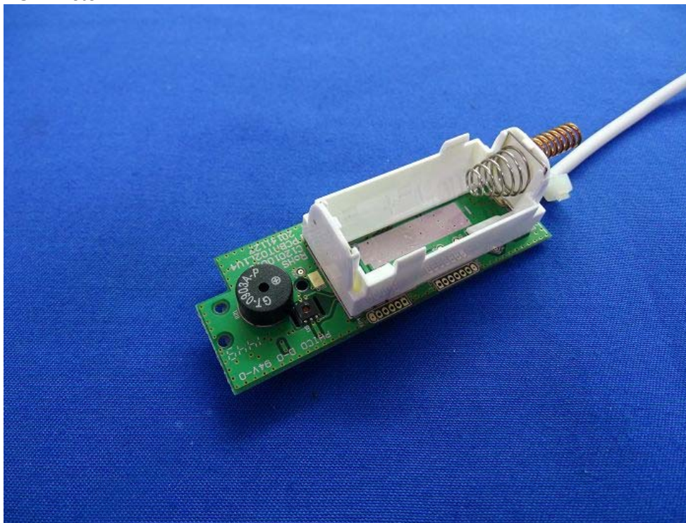
(13) EUT Photo
