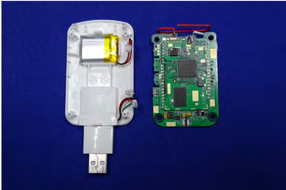
(8) EUT Photo
