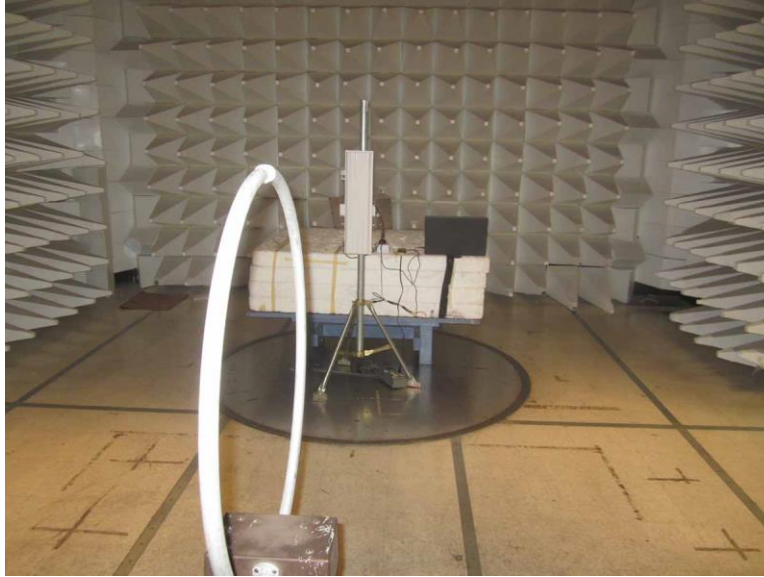
9kHz-30MHz, Perpendicular
