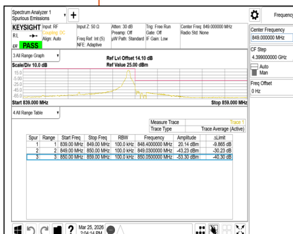
Band26 10MHz QPSK RB1 49 CH26990
