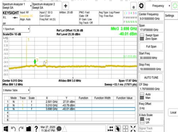
Band41_10MHz_DFT_s_OFDM_SCS30kHz_BPSK_RB1_1_CH501000upper 18G
