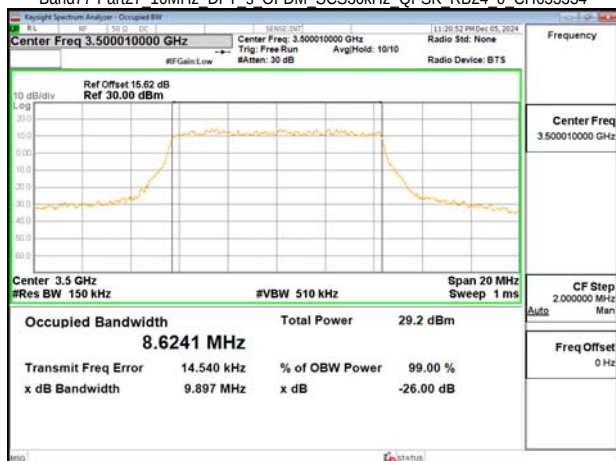
Band77-Part27 10MHz DFT s OFDM SCS30kHz QPSK RB24 0 CH633334
