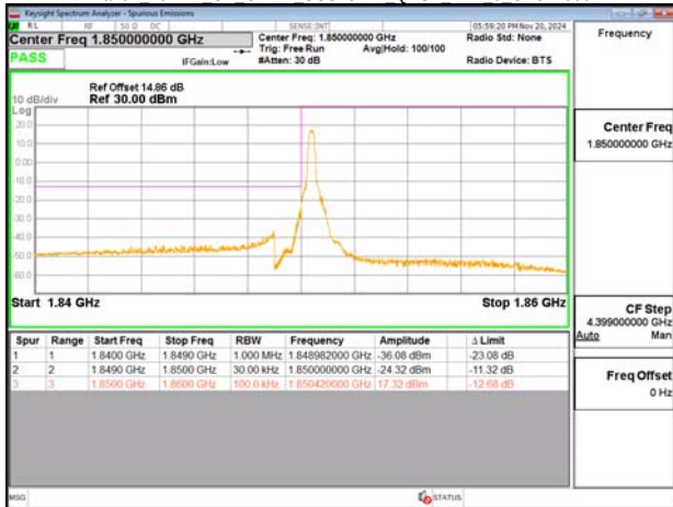
Band2 10MHz CP OFDM SCS15kHz QPSK RB52 0 CH371000
