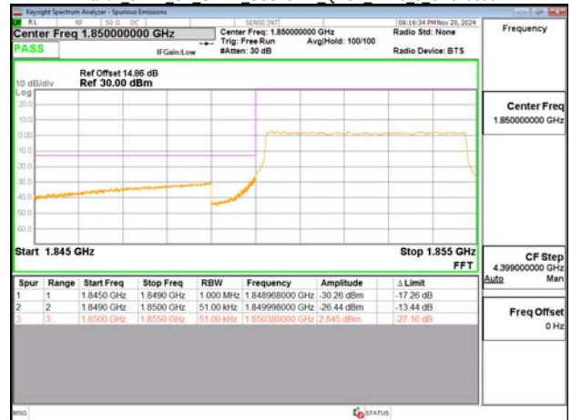
Band2 5MHz CP OFDM SCS15kHz QPSK RB25 0 CH370500
