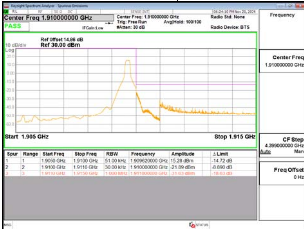
Band2 5MHz CP OFDM SCS15kHz QPSK RB25 0 CH381500
