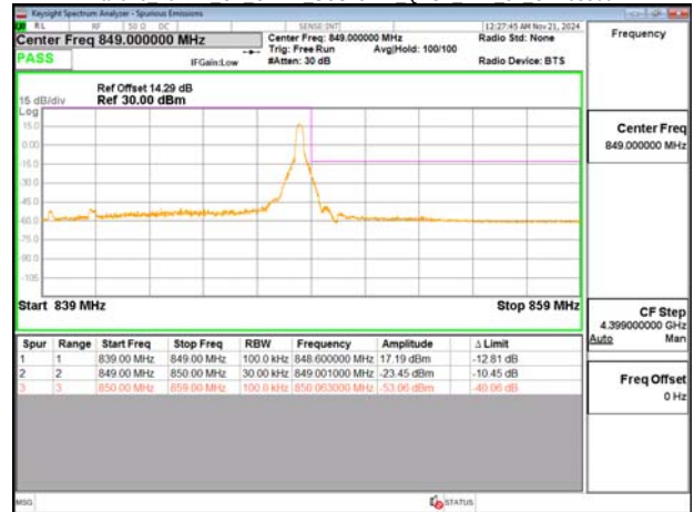
Band26 10MHz CP OFDM SCS15kHz QPSK RB52 0 CH168800
