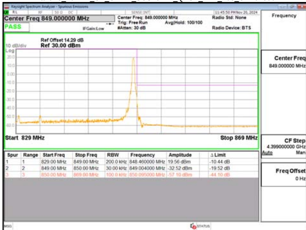
Band26 20MHz CP OFDM SCS15kHz QPSK RB1_105 CH167800
