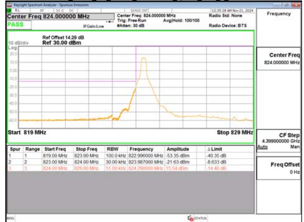
Band26 5MHz CP_OFDM SCS15kHz QPSK RB1 0 CH165300
