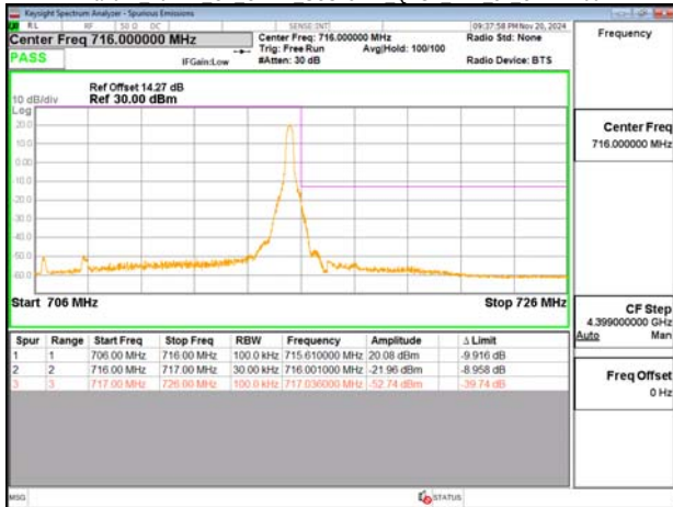
Band12 10MHz CP OFDM SCS15kHz QPSK RB52 0 CH142200
