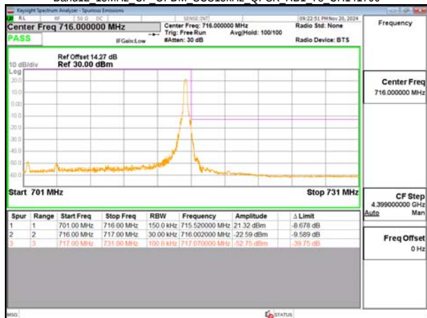
Band12 15MHz CP OFDM SCS15kHz QPSK RB1 78 CH141700
