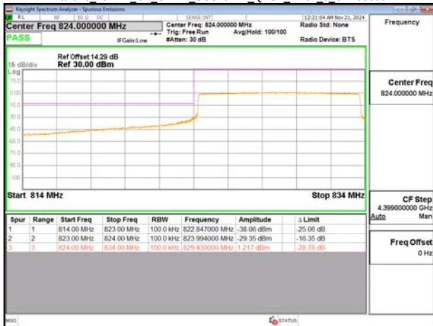
Band26 10MHz CP OFDM SCS15kHz QPSK RB52 0 CH165800
