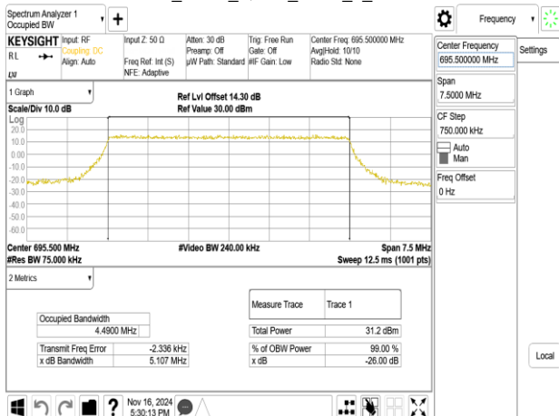
Band71_5MHz_QPSK_RB25_0_CH133447
