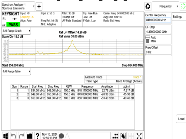
Band26_15MHz_QPSK_RB1_74_CH26965
