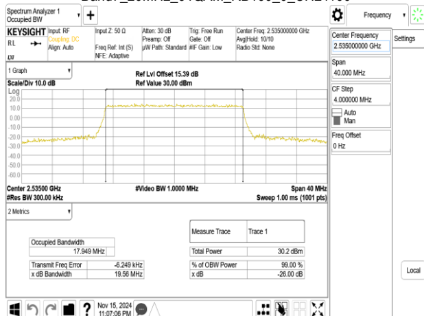
Band7_20MHz_256QAM_RB100_0_CH21100
