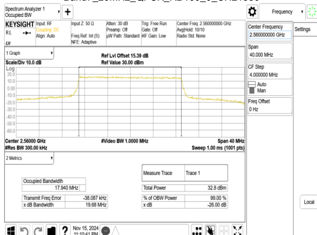
Band7_20MHz_QPSK_RB100_0_CH21350
