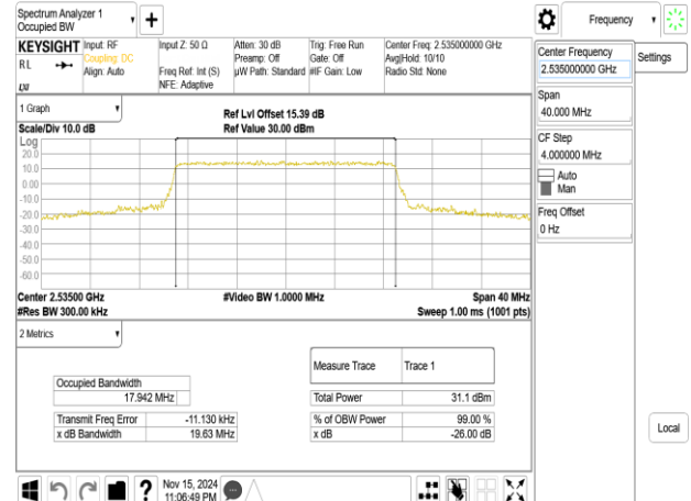
Band7_20MHz_16QAM_RB100_0_CH21100
