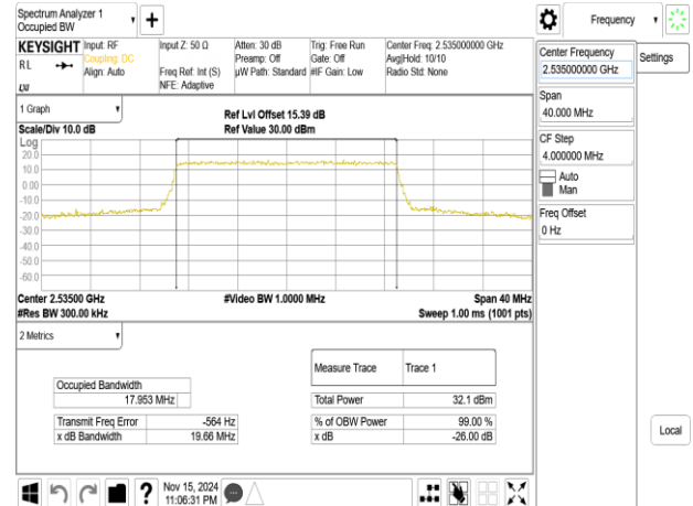
Band7_20MHz_16QAM_RB100_0_CH21100
