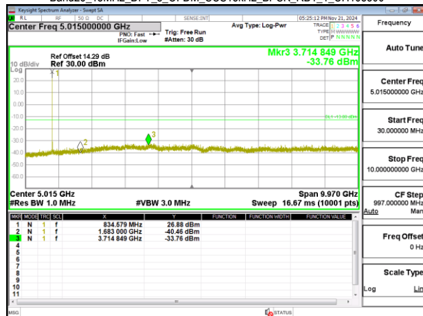
Band26_15MHz_DFT_s_OFDM_SCS15kHz_BPSK_RB1_1_CH168300
