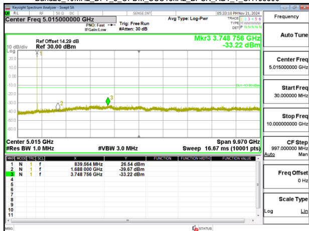
Band26_10MHz_DFT_s_OFDM_SCS15kHz_BPSK_RB1_1_CH168800
