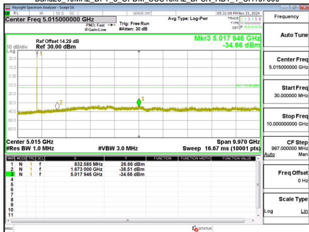
Band26_10MHz_DFT_s_OFDM_SCS15kHz_BPSK_RB1_1_CH168800
