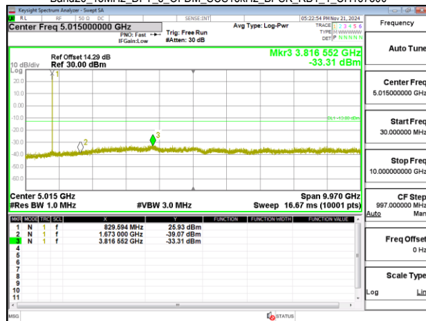
Band26_15MHz_DFT_s_OFDM_SCS15kHz_BPSK_RB1_1_CH168300
