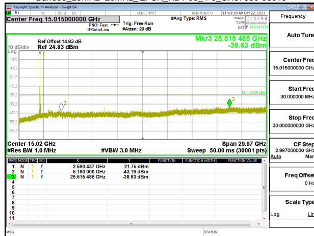
Band38_20MHz+20MHz_QPSK_RB1-99_1-0_CH37901-38099
