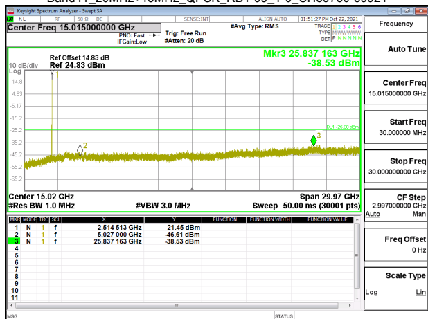
Band41_20MHz+15MHz_QPSK_RB1-99_1-0_CH40546-40717
