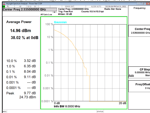
Band7_20MHz+15MHz_64QAM_RB100-0+RB75-0_CH21026+CH21197
