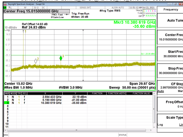
Band38_20MHz+20MHz_QPSK_RB1-99_1-0_CH37952-38150
