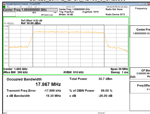
Band25_20MHz_QPSK_RB100_0_CH26590
