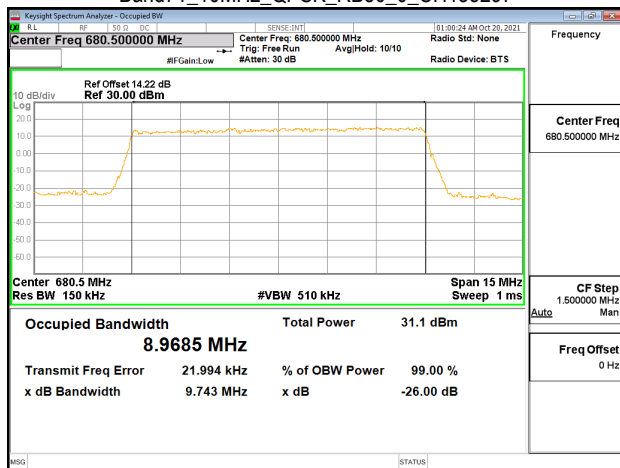
Band71_10MHz_QPSK_RB50_0_CH133422
