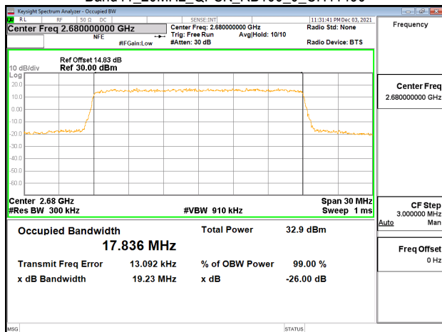
Band41_20MHz_QPSK_RB100_0_CH41490
