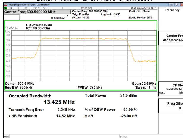
Band71_15MHz_QPSK_RB75_0_CH133397
