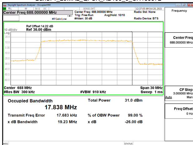
Band71_20MHz_QPSK_RB100_0_CH133372
