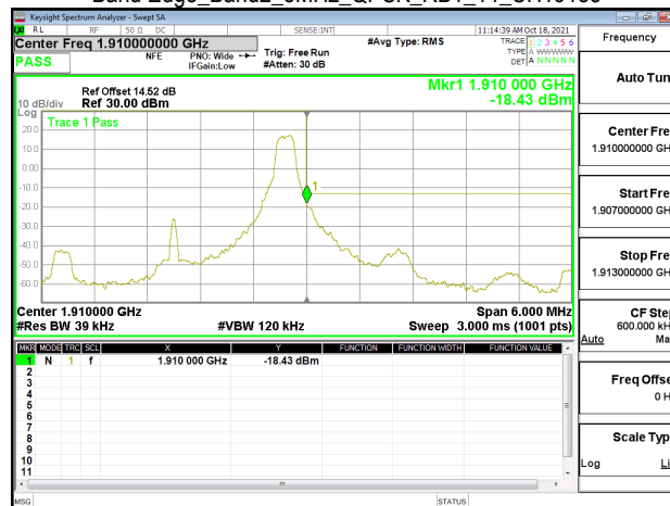
Band Edge_Band2_3MHz_QPSK_RB1_14_CH19185
