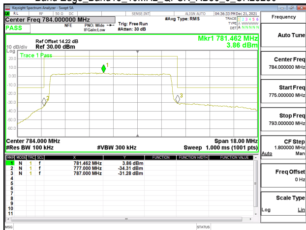
Band Edge_Band13_10MHz_QPSK_RB50_0_CH23230
