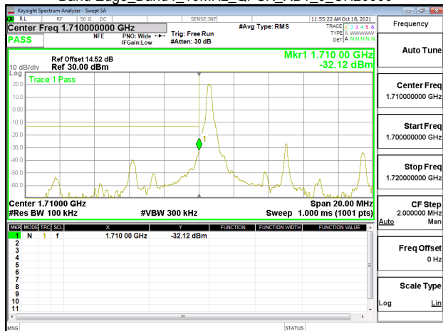
Band Edge_Band4_10MHz_QPSK_RB1_49_CH20350
