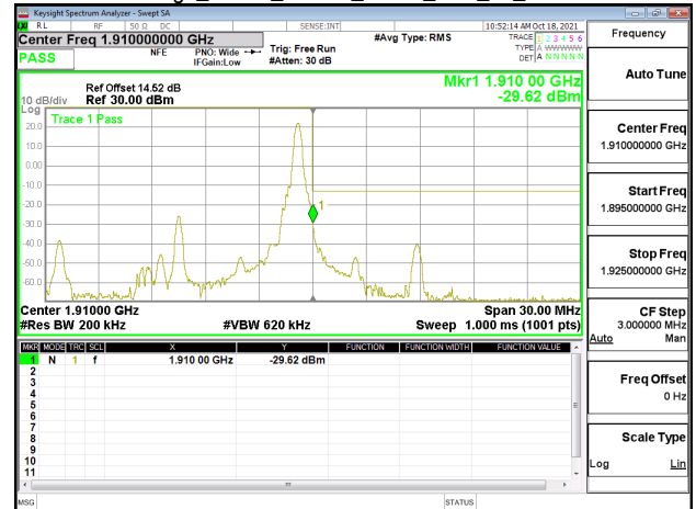
Band Edge_Band2_15MHz_QPSK_RB1_74_CH19125
