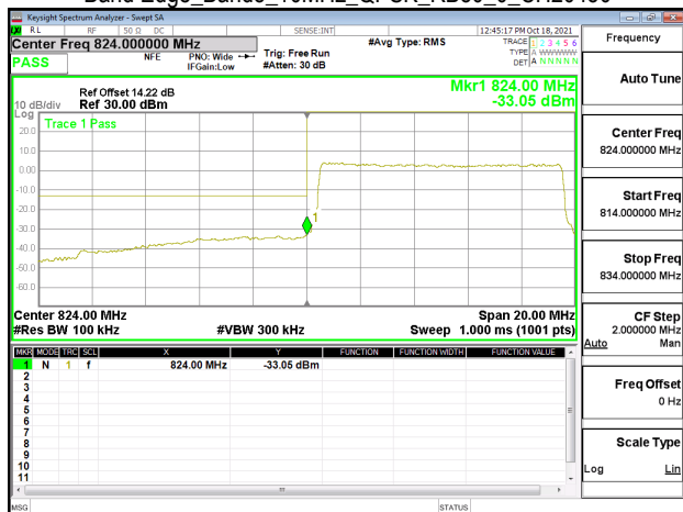
Band Edge_Band5_10MHz_QPSK_RB50_0_CH20450
