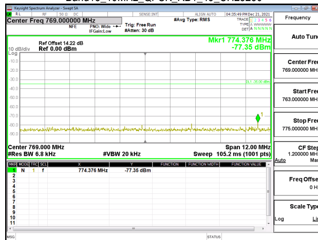
Band13_10MHz_QPSK_RB50_0_CH23230
