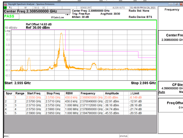
Emission Mask_Band7_20MHz_QPSK_RB1_99_CH21350
