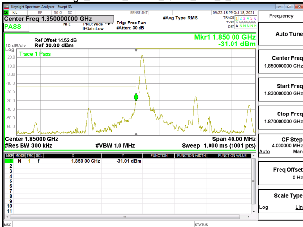
Band Edge_Band25_20MHz_QPSK_RB1_0_CH26140
