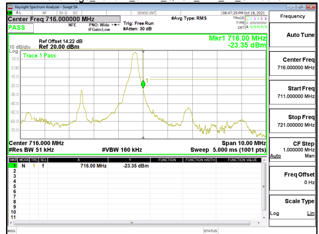
Band Edge_Band17_5MHz_QPSK_RB1_24_CH23825
