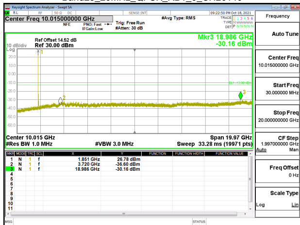
Band25_20MHz_QPSK_RB1_0_CH26140
