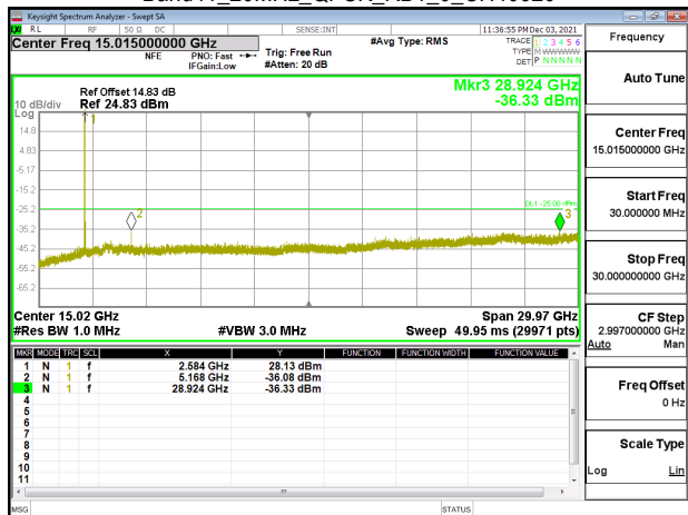
Band41_20MHz_QPSK_RB1_0_CH41490
