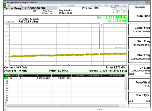
Band30_10MHz_QPSK_RB1_0_CH27710_2
