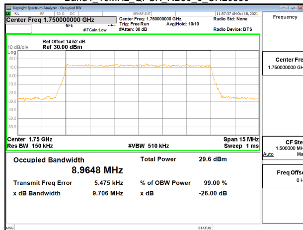
Band4_10MHz_QPSK_RB50_0_CH20350
