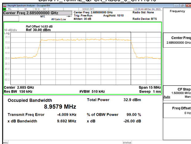
Band41_10MHz_QPSK_RB50_0_CH41540
