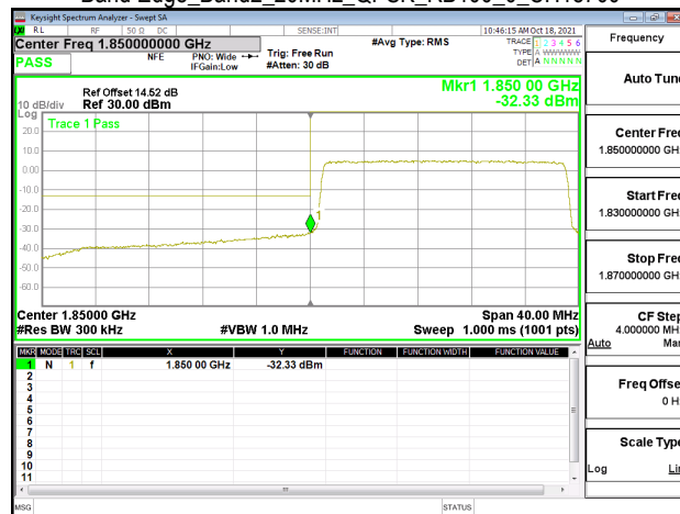
Band Edge_Band2_20MHz_QPSK_RB100_0_CH19100
