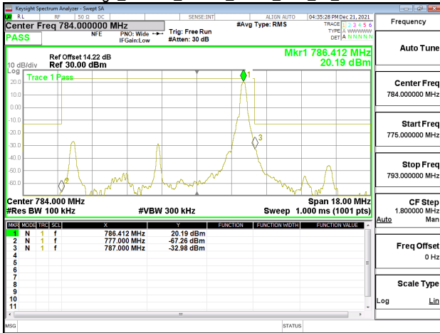
Band Edge_Band13_10MHz_QPSK_RB50_0_CH23230
