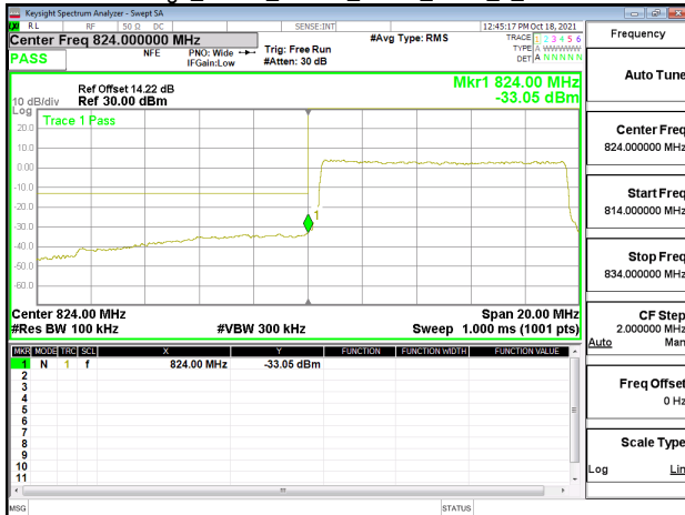
Band Edge_Band5_10MHz_QPSK_RB50_0_CH20450
