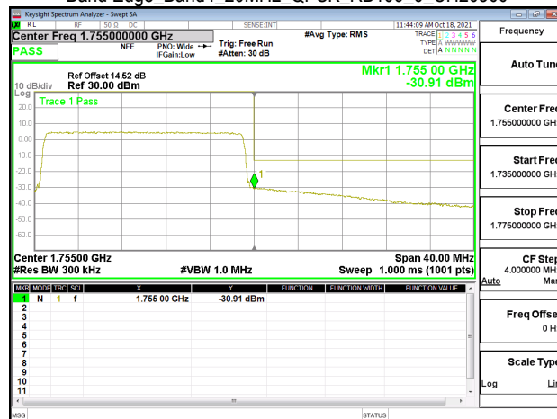
Band Edge_Band4_20MHz_QPSK_RB100_0_CH20300
