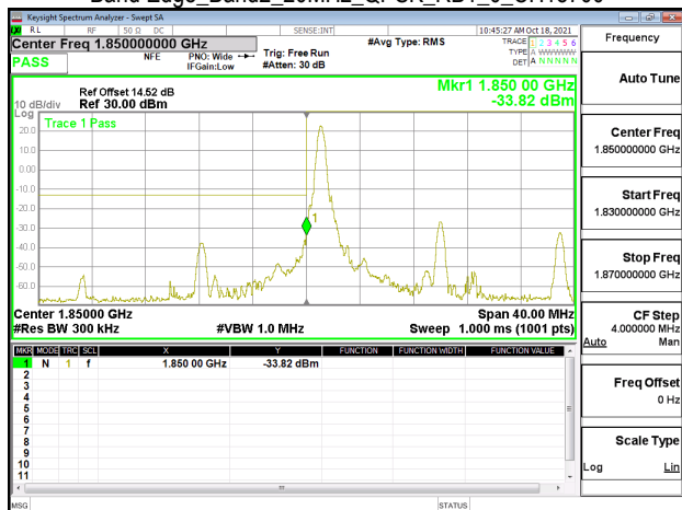
Band Edge_Band2_20MHz_QPSK_RB1_0_CH18700
