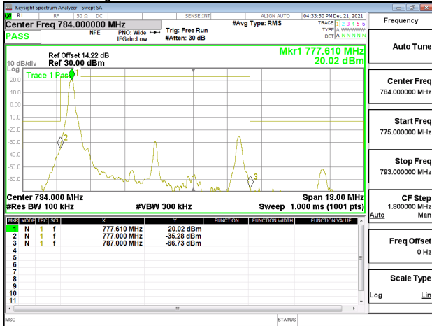
Band Edge_Band13_10MHz_QPSK_RB1_49_CH23230
