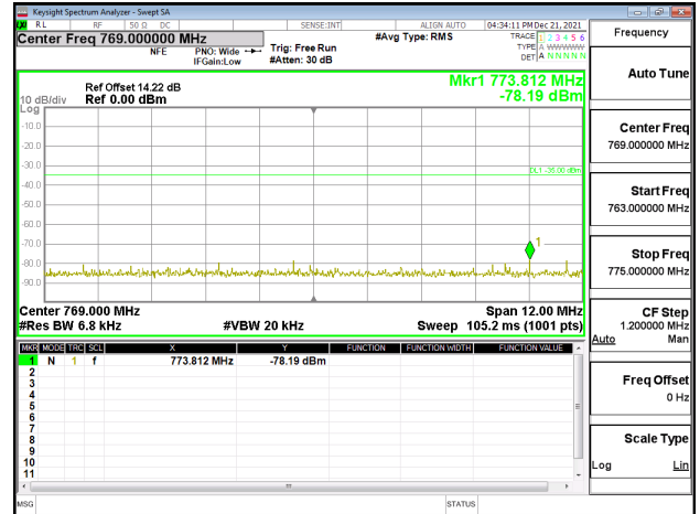
Band13_10MHz_QPSK_RB1_49_CH23230
