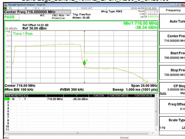
Band Edge_Band12_10MHz_QPSK_RB50_0_CH23130
