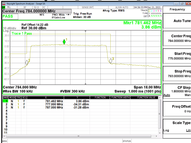
Band Edge_Band13_10MHz_QPSK_RB50_0_CH23230
