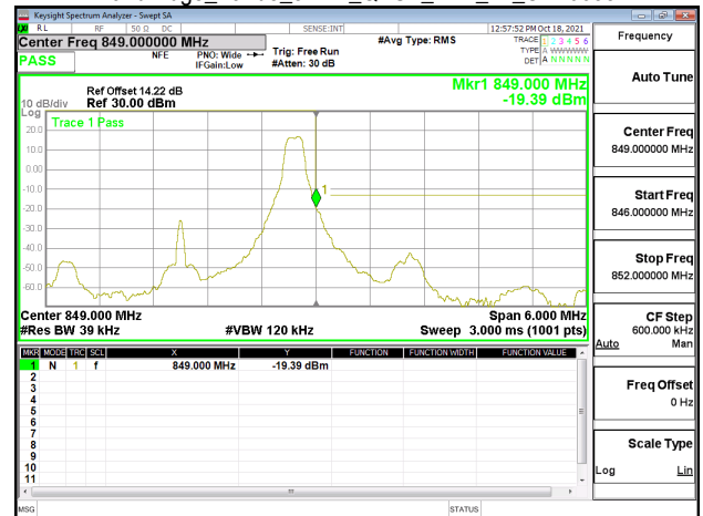
Band Edge_Band5_3MHz_QPSK_RB1_14_CH20635
