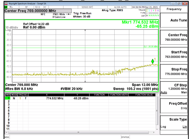
Band13_10MHz_QPSK_RB50_0_CH23230
