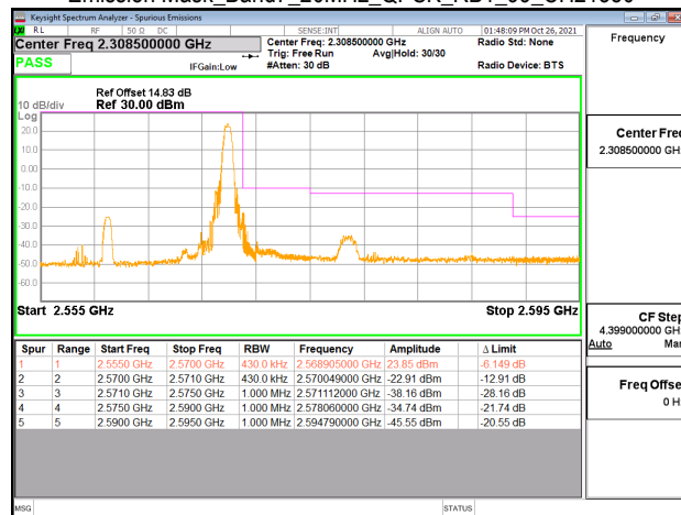
Emission Mask_Band7_20MHz_QPSK_RB1_99_CH21350
