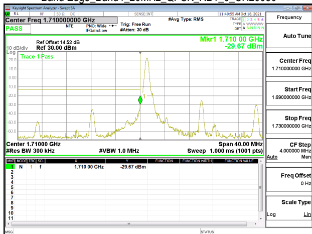
Band Edge_Band4_20MHz_QPSK_RB1_0_CH20050
