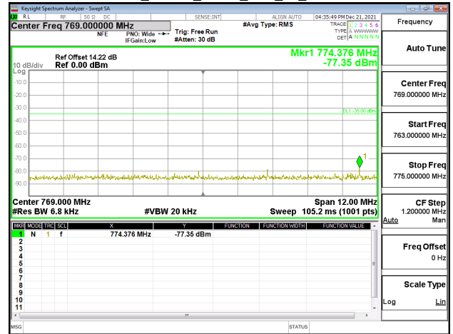
Band13_10MHz_QPSK_RB50_0_CH23230
