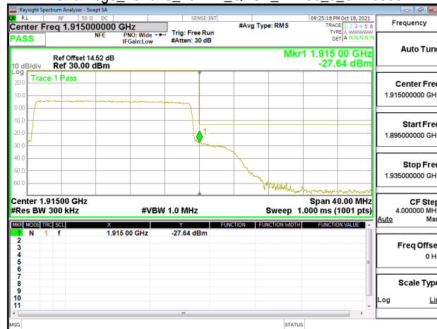
Band Edge_Band25_20MHz_QPSK_RB100_0_CH26590
