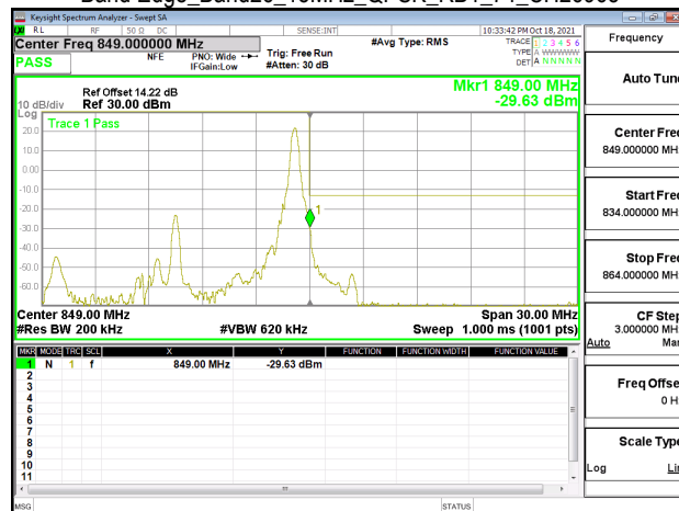
Band Edge_Band26_15MHz_QPSK_RB1_74_CH26965
