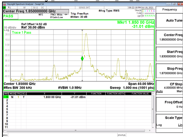
Band Edge_Band25_20MHz_QPSK_RB1_0_CH26140
