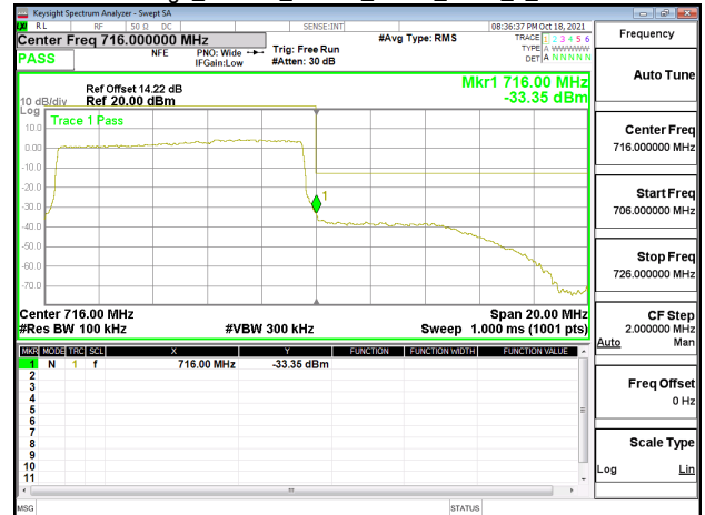
Band Edge_Band17_10MHz_QPSK_RB50_0_CH23800
