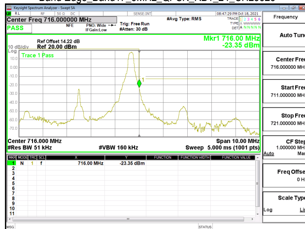
Band Edge_Band17_5MHz_QPSK_RB1_24_CH23825
