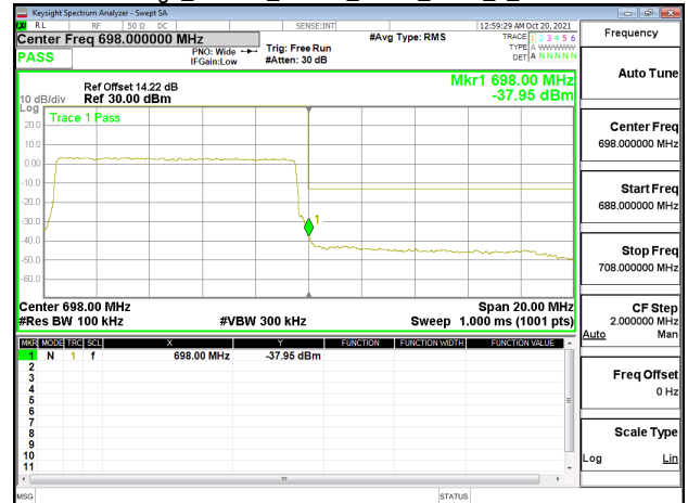
Band Edge_Band71_10MHz_QPSK_RB50_0_CH133422
