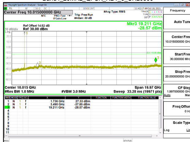
Band4_20MHz_QPSK_RB1_0_CH20300
