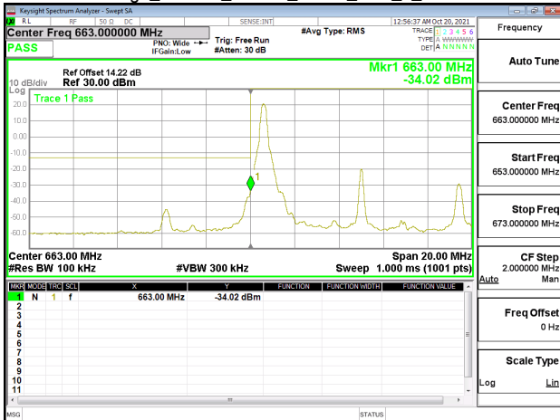
Band Edge_Band71_10MHz_QPSK_RB1_0_CH133172
