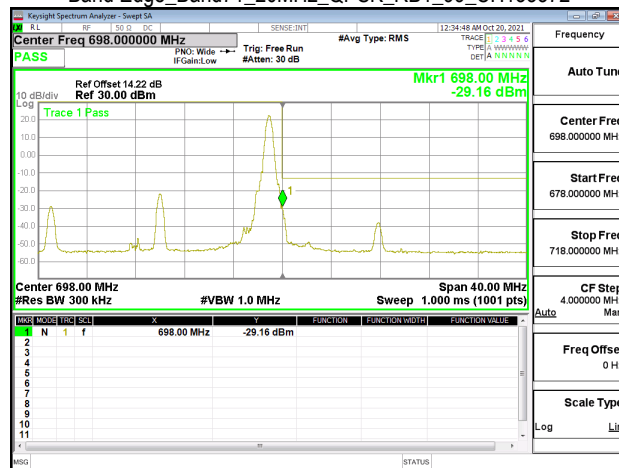
Band Edge_Band71_20MHz_QPSK_RB1_99_CH133372
