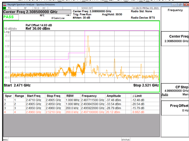
Emission Mask_Band41_20MHz_QPSK_RB1_99_CH41490
