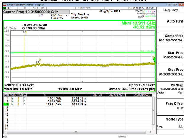
Band2_10MHz_QPSK_RB1_0_CH19150
