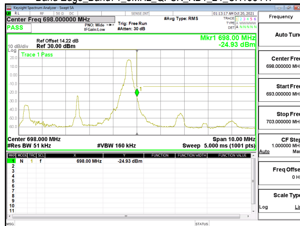
Band Edge_Band71_5MHz_QPSK_RB1_24_CH133447
