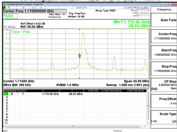
Band Edge_Band66_20MHz_QPSK_RB1_99_CH132572
