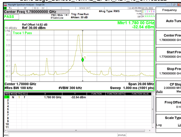
Band Edge_Band66_10MHz_QPSK_RB1_49_CH132622
