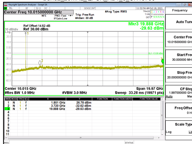
Band2_20MHz_QPSK_RB1_0_CH18900
