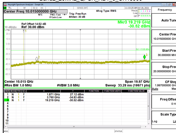
Band2_20MHz_QPSK_RB1_0_CH19100
