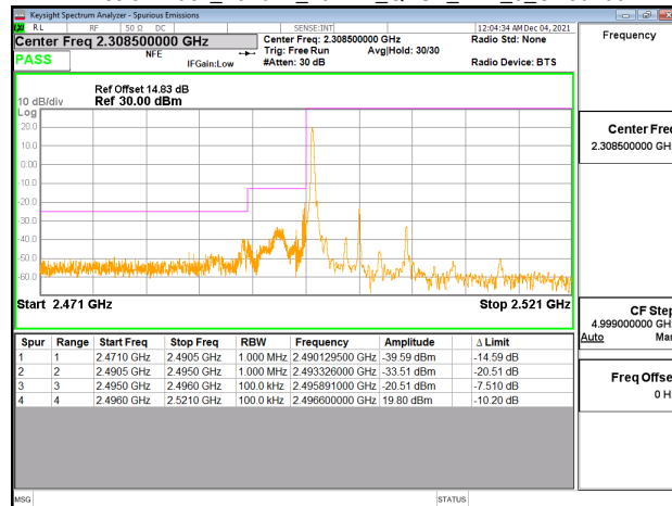
Emission Mask_Band41_10MHz_QPSK_RB1_49_CH41540
