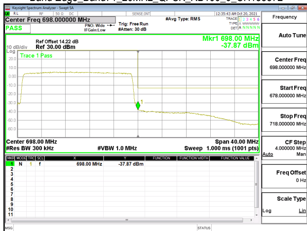
Band Edge_Band71_20MHz_QPSK_RB100_0_CH133372
