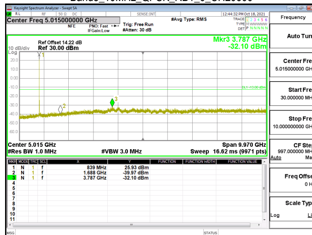
Band5_10MHz_QPSK_RB1_0_CH20600
