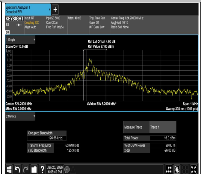
B26(824-849)-15KHz-QPSK-26915-1RB#0-PASS
