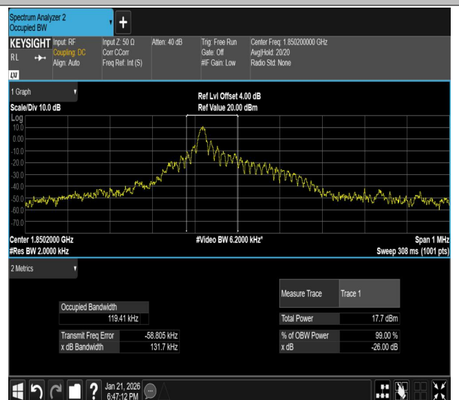
Band25-15KHz-QPSK-26365-1RB#0-PASS
