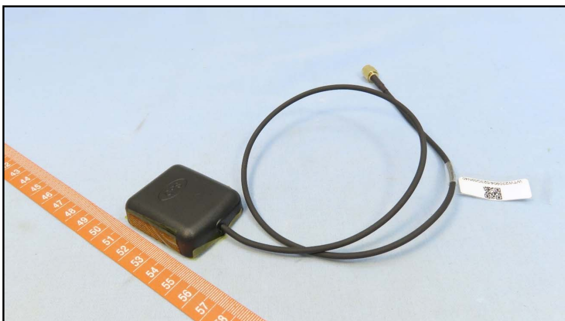
GPS Antenna
