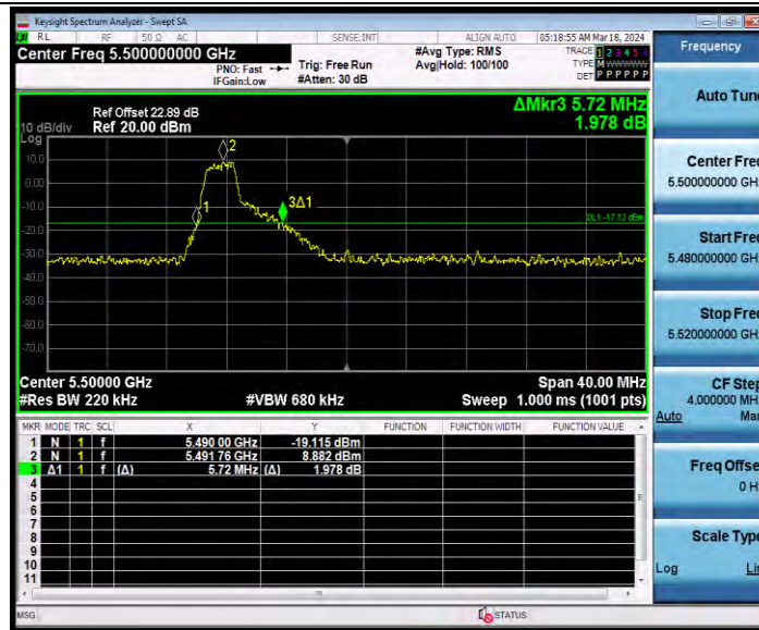
11AX20SISO_Ant2_5500_52Tone_RU37
