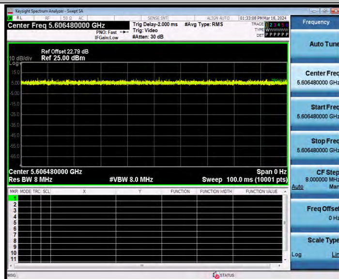
11AX80MIMO_Ant1_5610_996Tone_RU67
