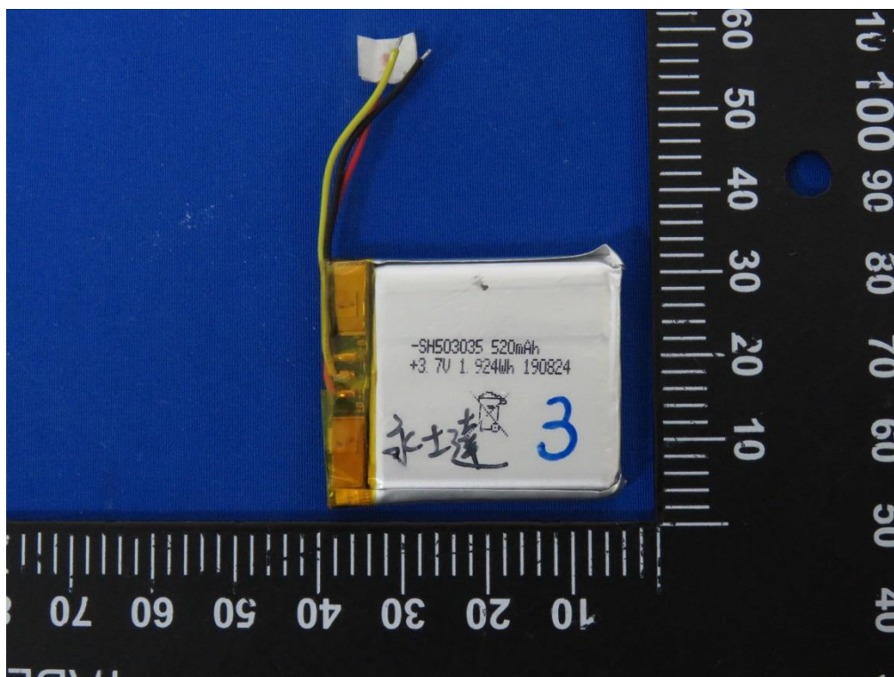
Battery: SH503035
