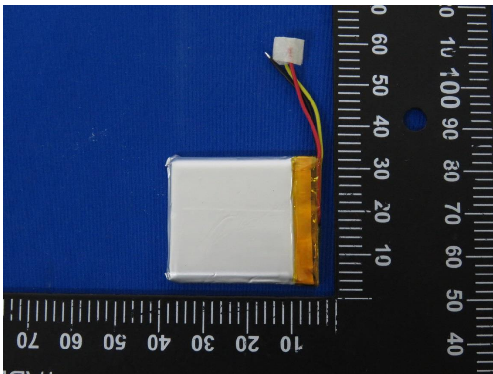
Battery: SH503035
