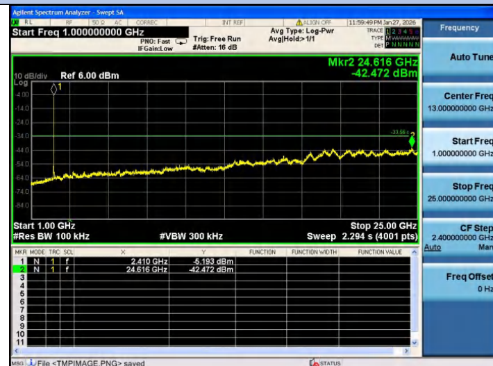
IEEE 802.11b_Ant1_CH01 2412MHz 1-25GHz
