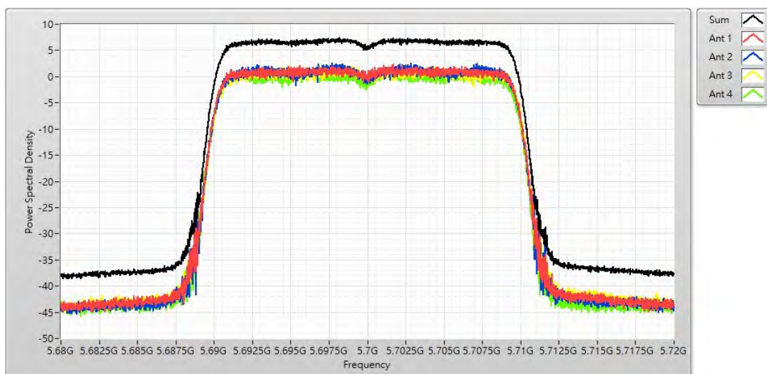
Channel 140 (5700MHz)
