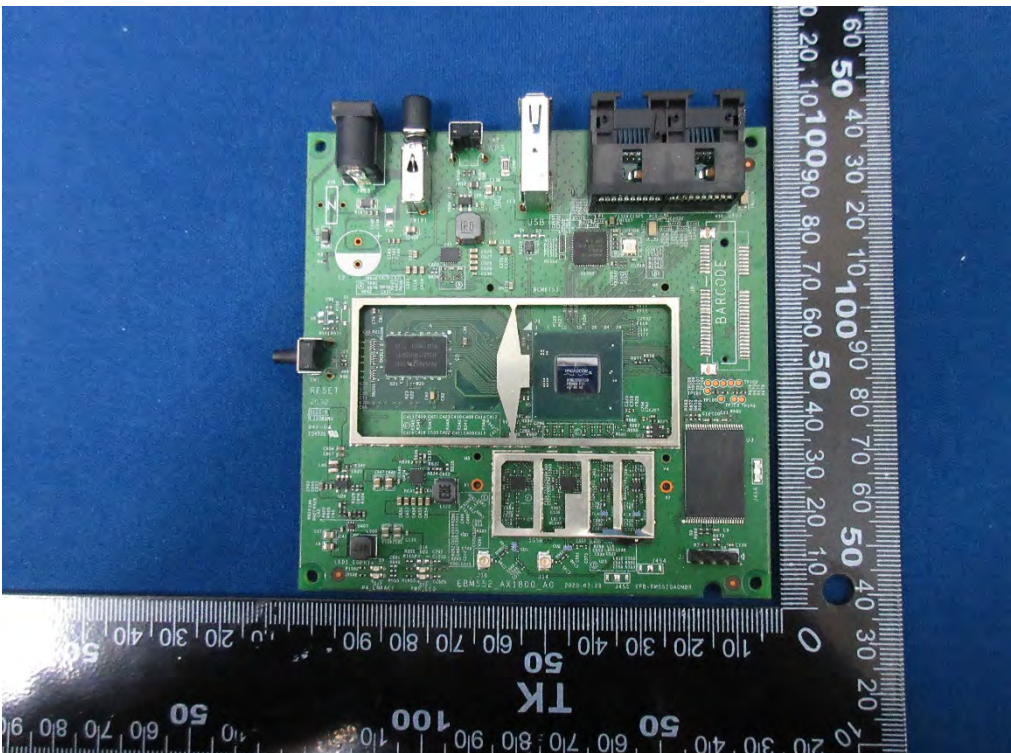
(9) EUT Photo
