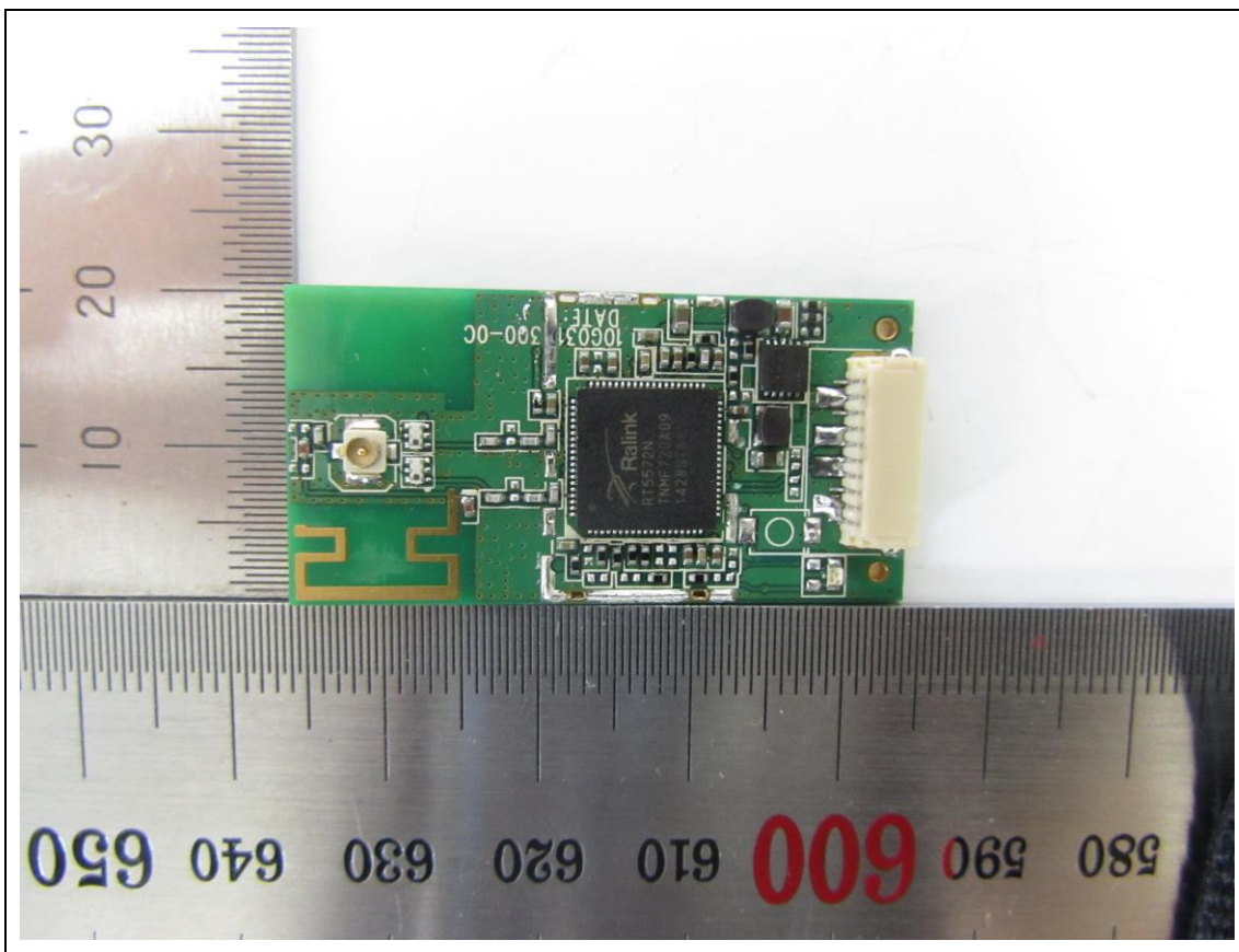
<Module>
