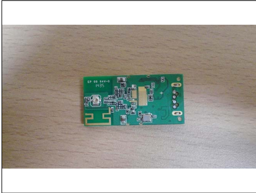
RF Module(Bottom)
