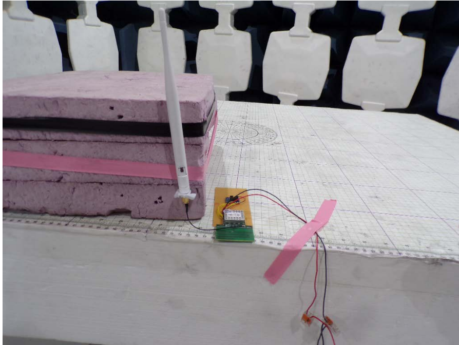
Module: Z-Axis External Antenna: Vertical
