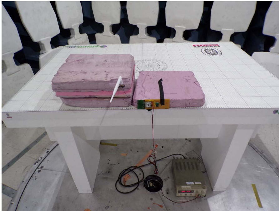
Module: Y-Axis External Antenna: Horizontal
