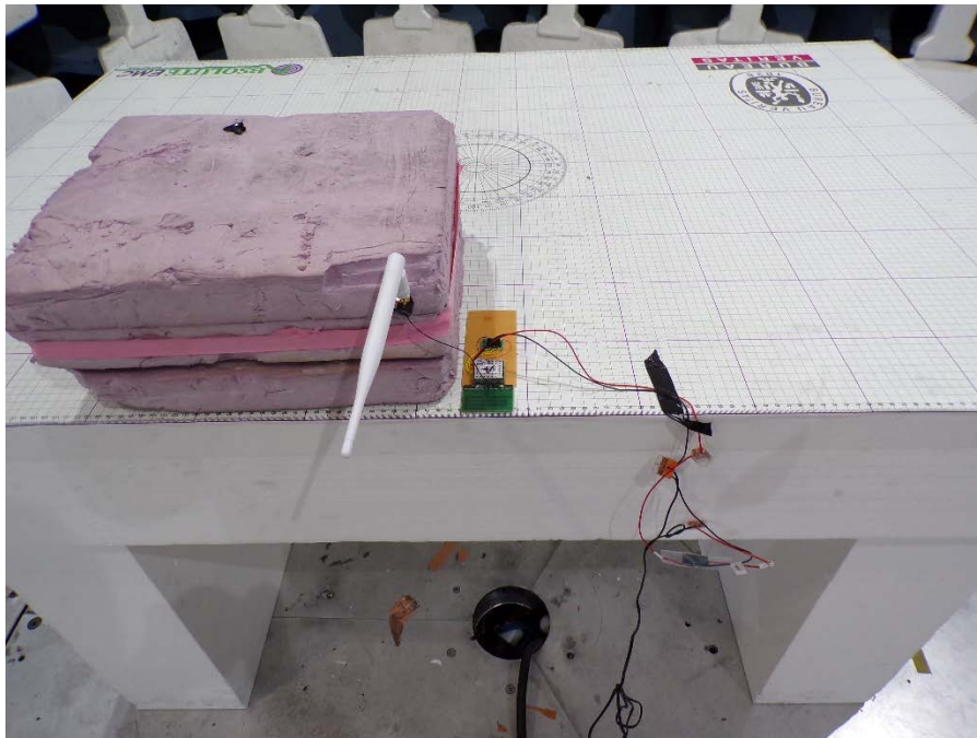
Module: Z-Axis External Antenna: Horizontal
