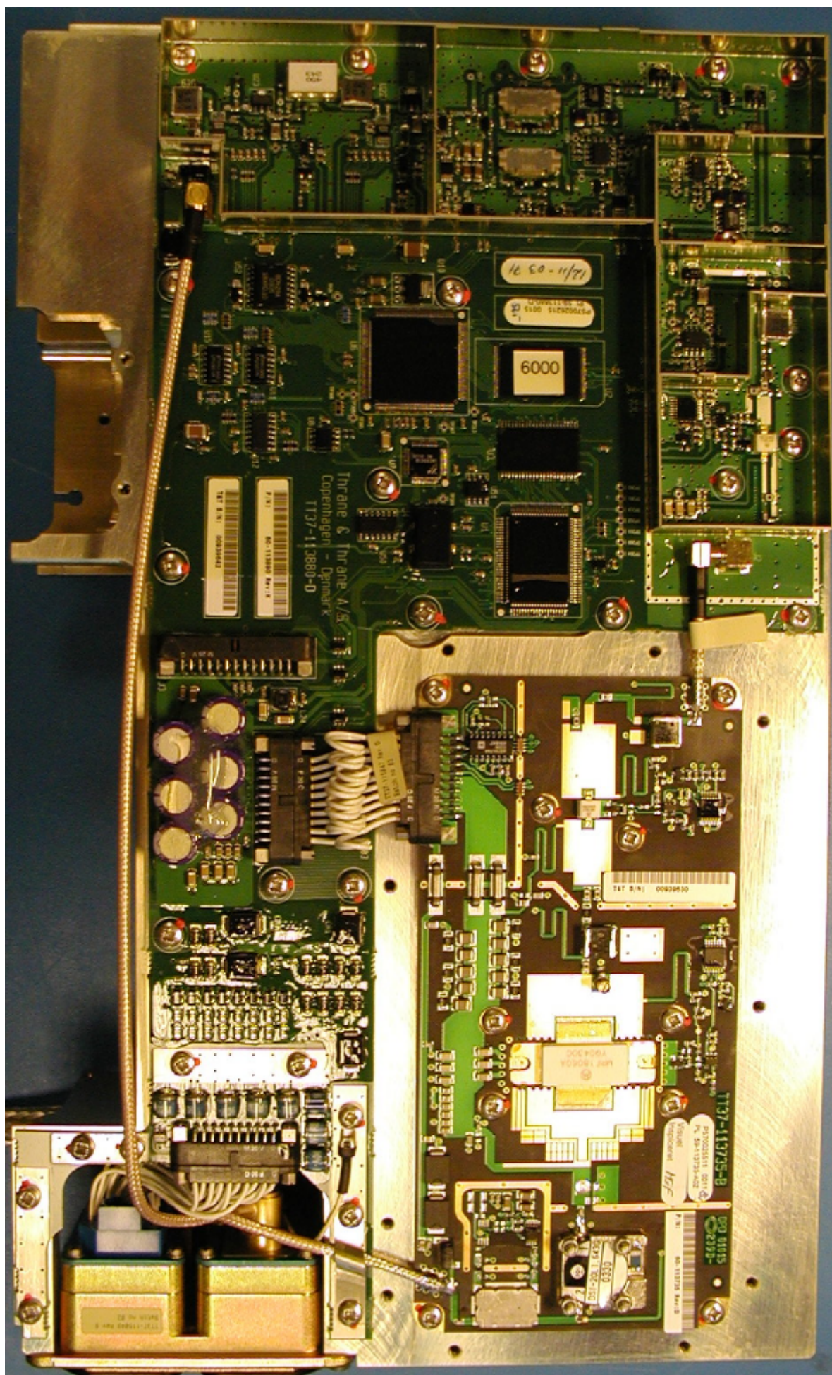
TT-5014A HPA Righ: TT93-113735 Left: TT93-113880
