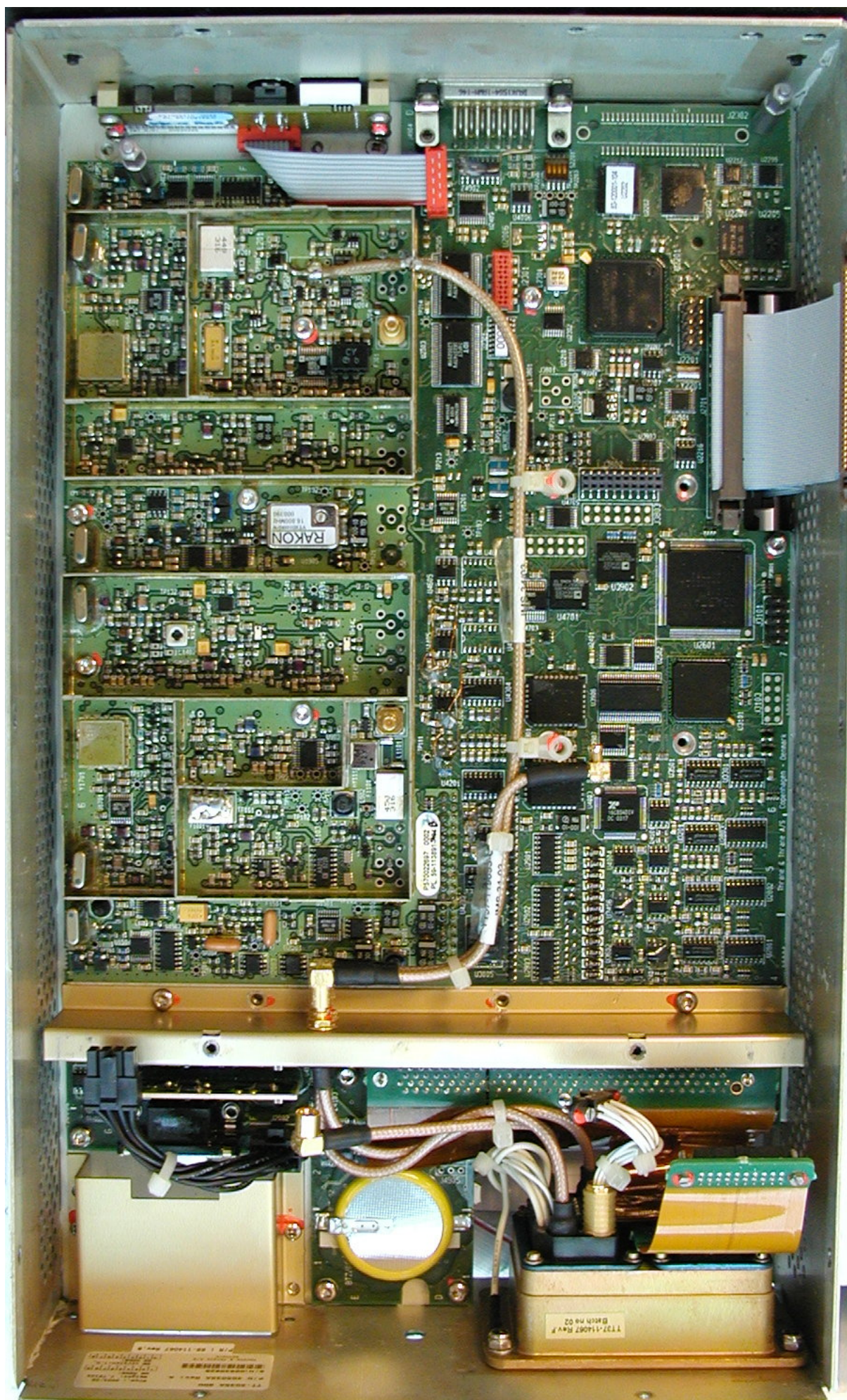
TT-5035A SDU
