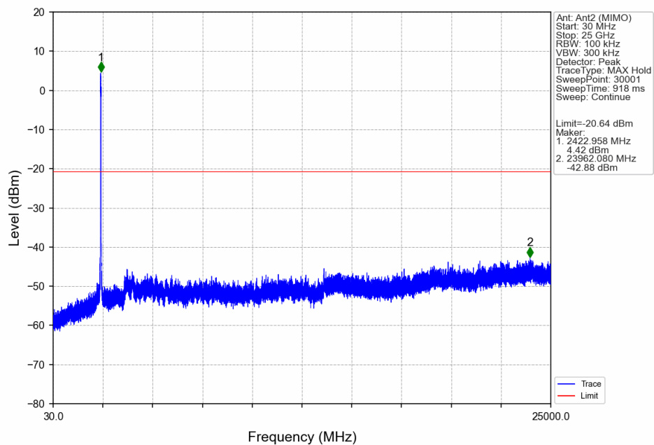
802.11be(EHT40)_LCH_2422MHz_SU_/_Ant2 (MIMO)_NTNV
