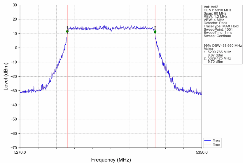
802.11be(EHT40)_HCH_5310MHz_SU_/_Ant2_NTNV
