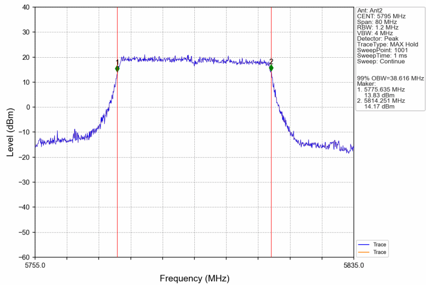
802.11be(EHT40)_HCH_5795MHz_SU_/_Ant2_NTNV
