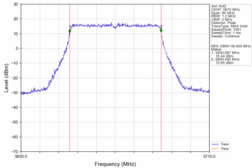
802.11be(EHT40)_HCH_5670MHz_SU_/_Ant2_NTNV
