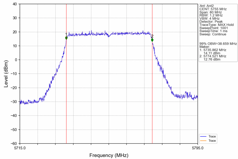
802.11be(EHT40)_LCH_5755MHz_SU_/_Ant2_NTNV
