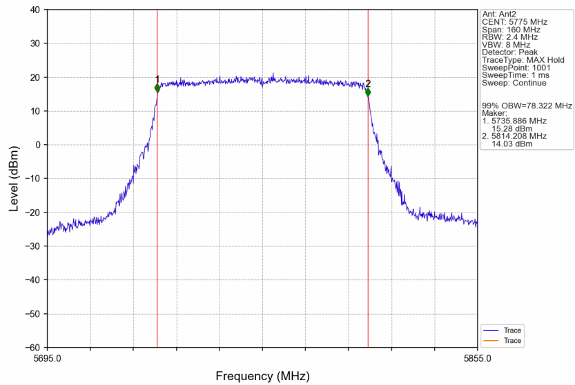
802.11be(EHT80)_MCH_5775MHz_SU_/_Ant2_NTNV
