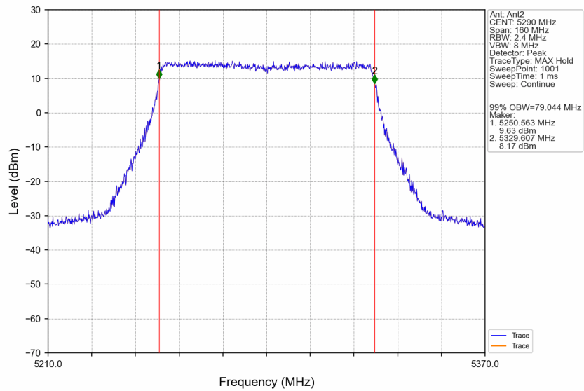
802.11be(EHT80)_MCH_5290MHz_SU_/_Ant2_NTNV
