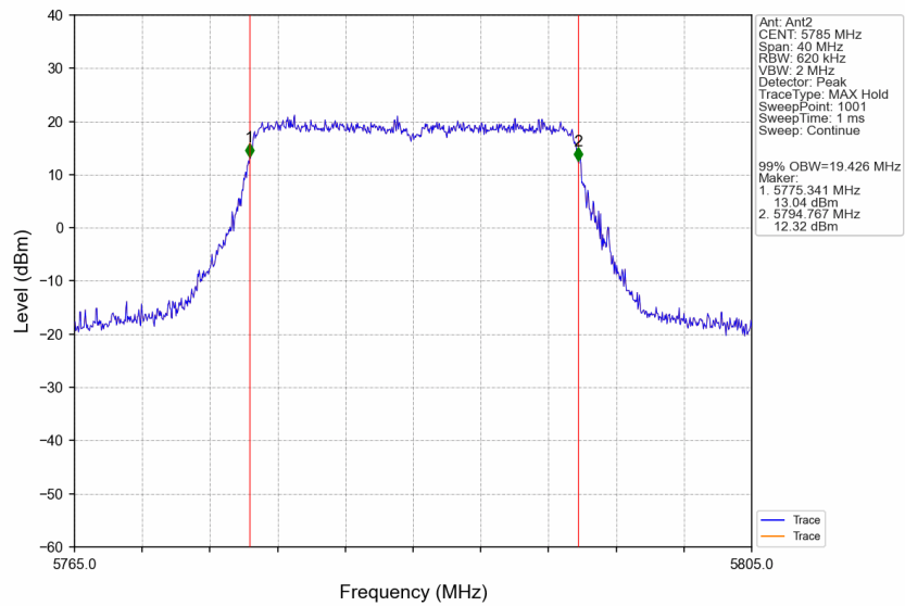
802.11be(EHT20)_MCH_5785MHz_SU_/_Ant2_NTNV
