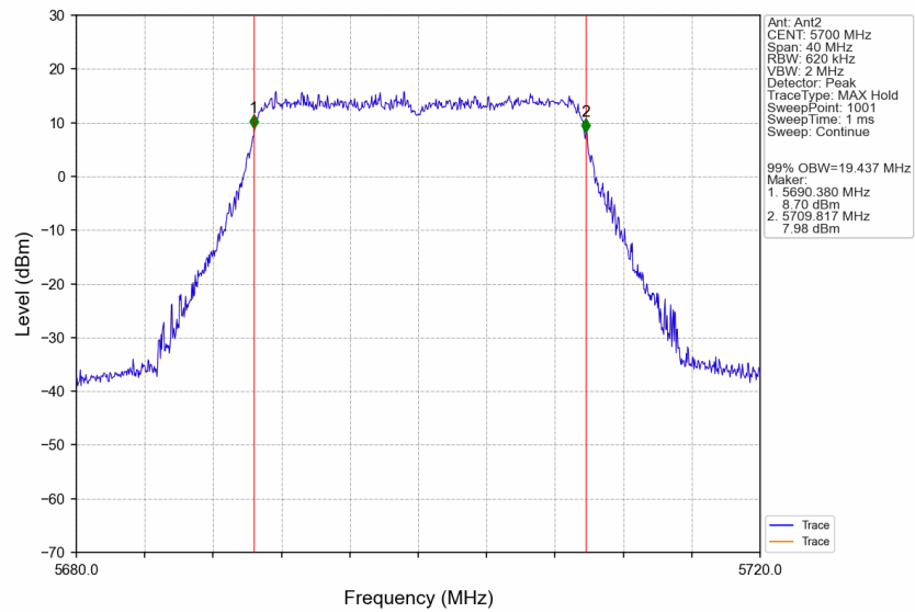
802.11be(EHT20)_HCH_5700MHz_SU_/_Ant2_NTNV
